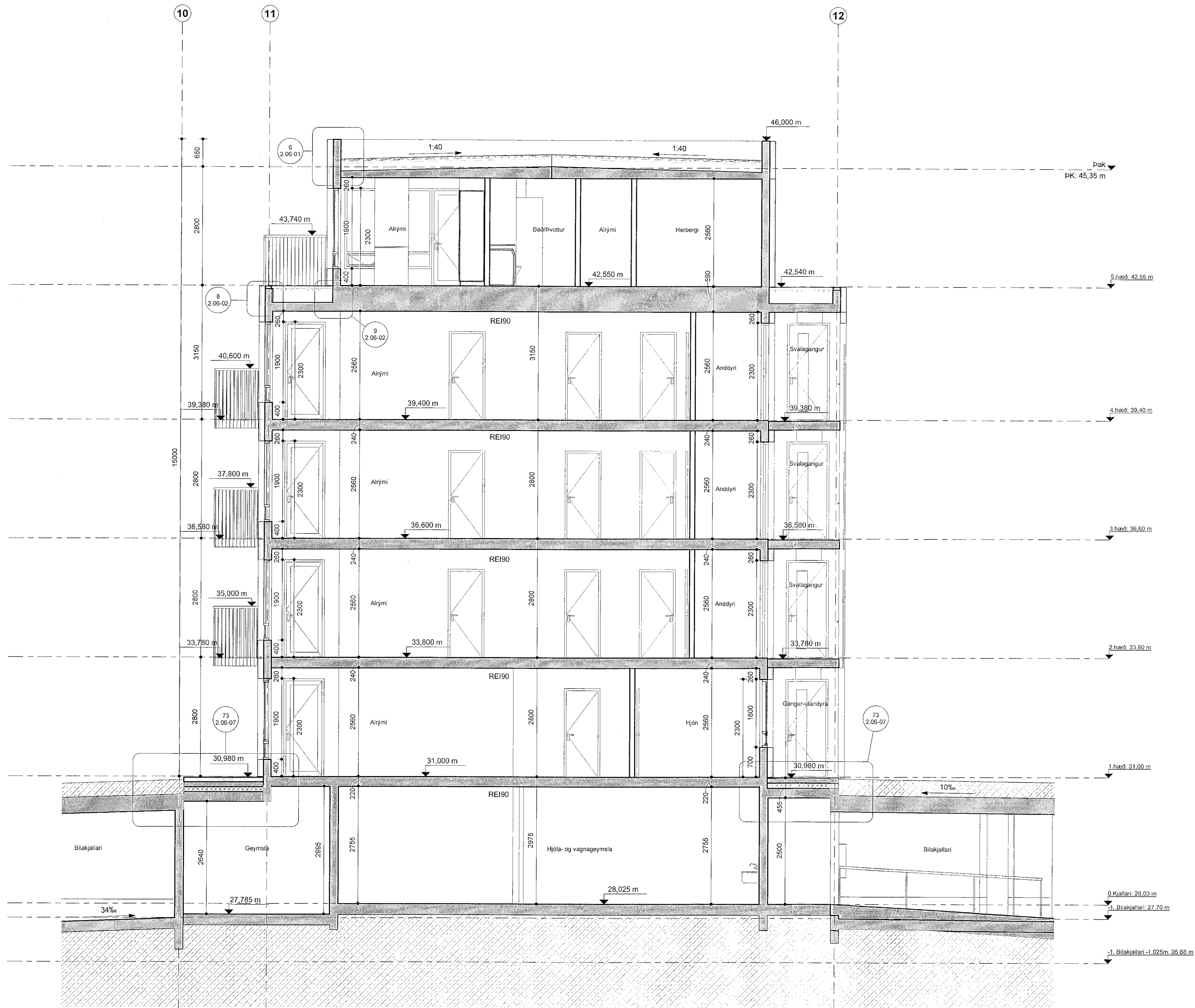
Áshamar 26 mhl.06 - snið n-n mkv: 1 : 50
