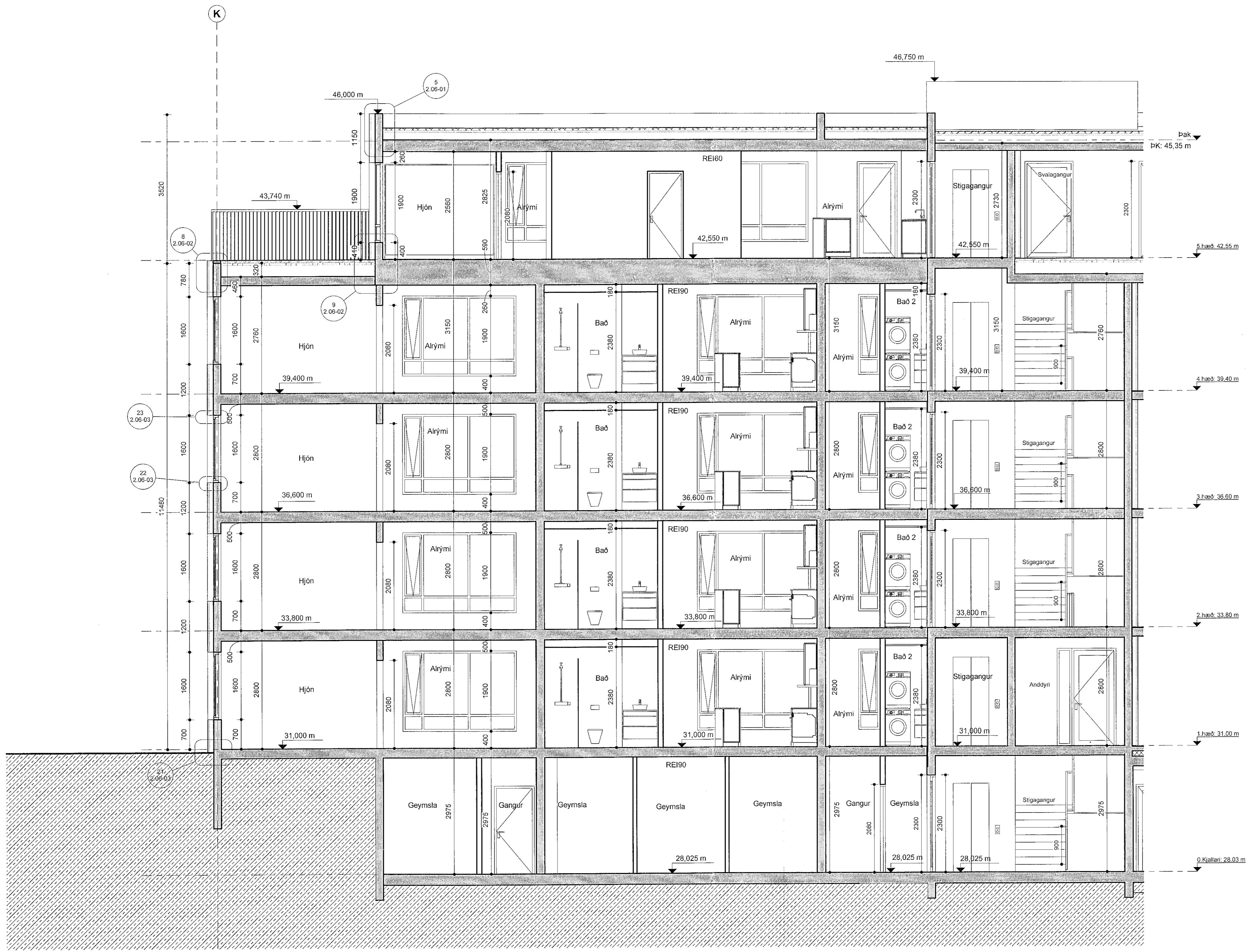
Áshamar 26 mhl.06 - snið i-i - hluti 1 mkv: 1 : 50
