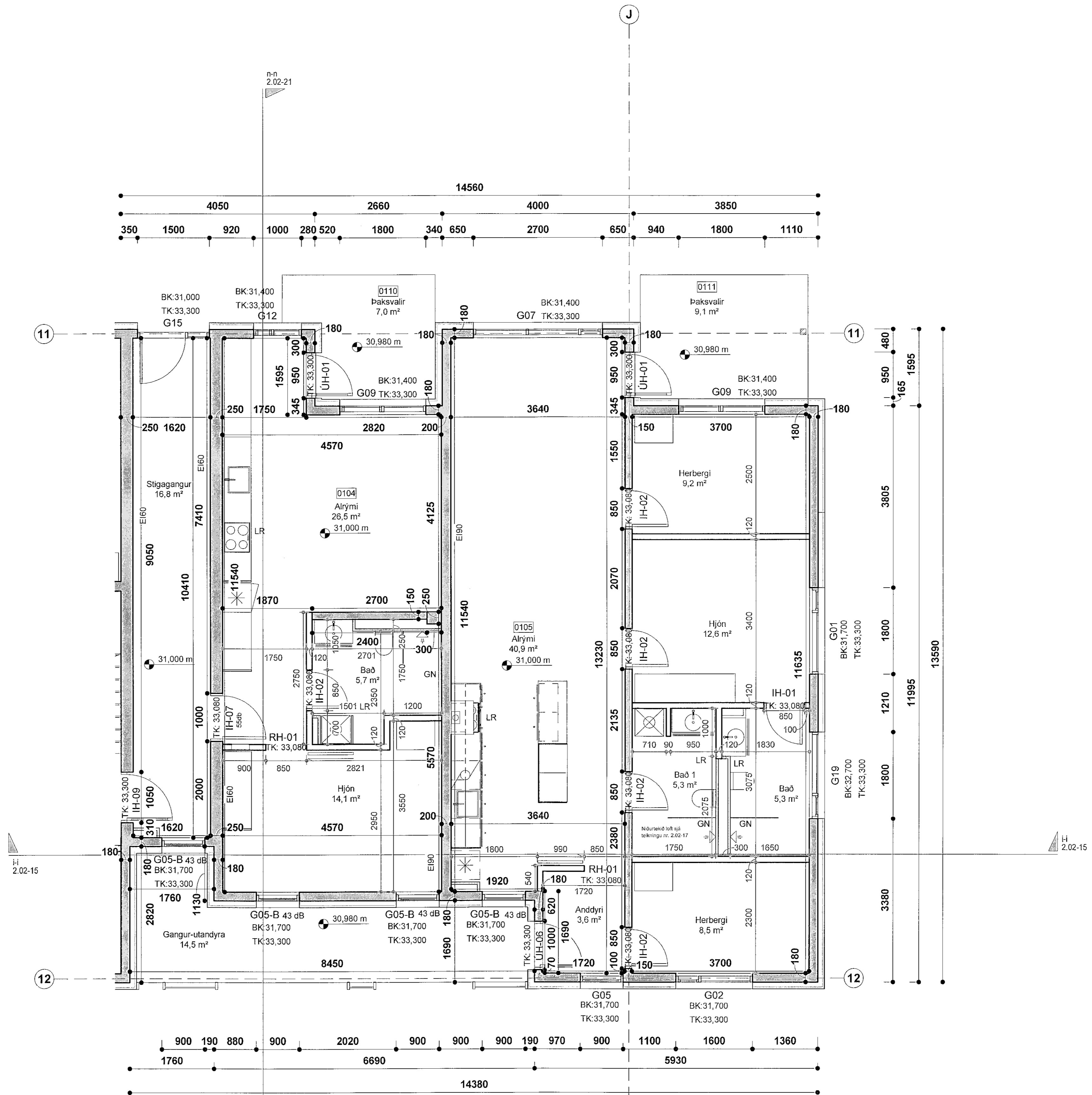
Ashamar 26 - 1.hæð - hluti 2 mkv: 1 : 50
