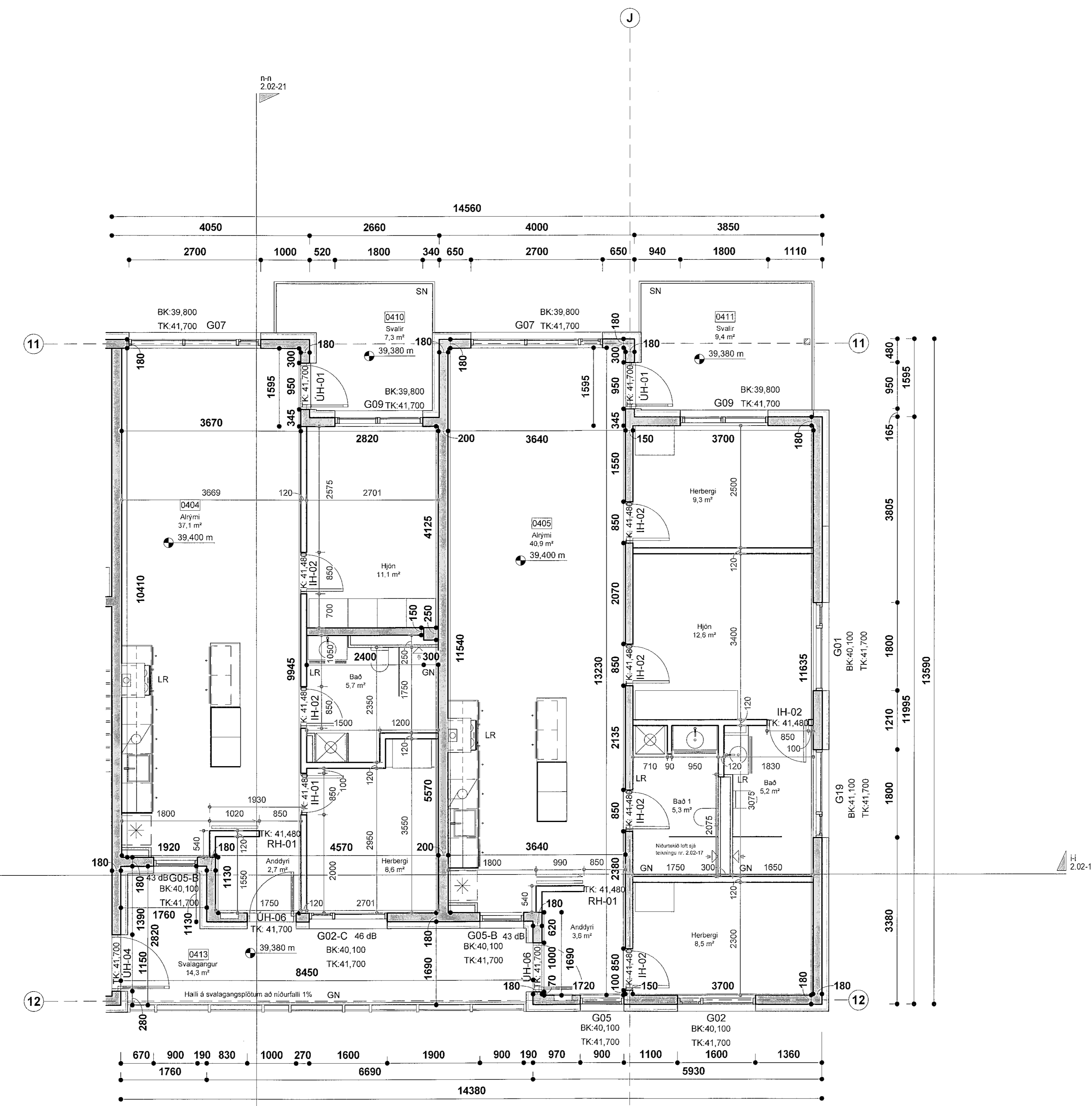
Áshamar 26 - 4.hæð - hluti 2 mkv: 1 : 50
