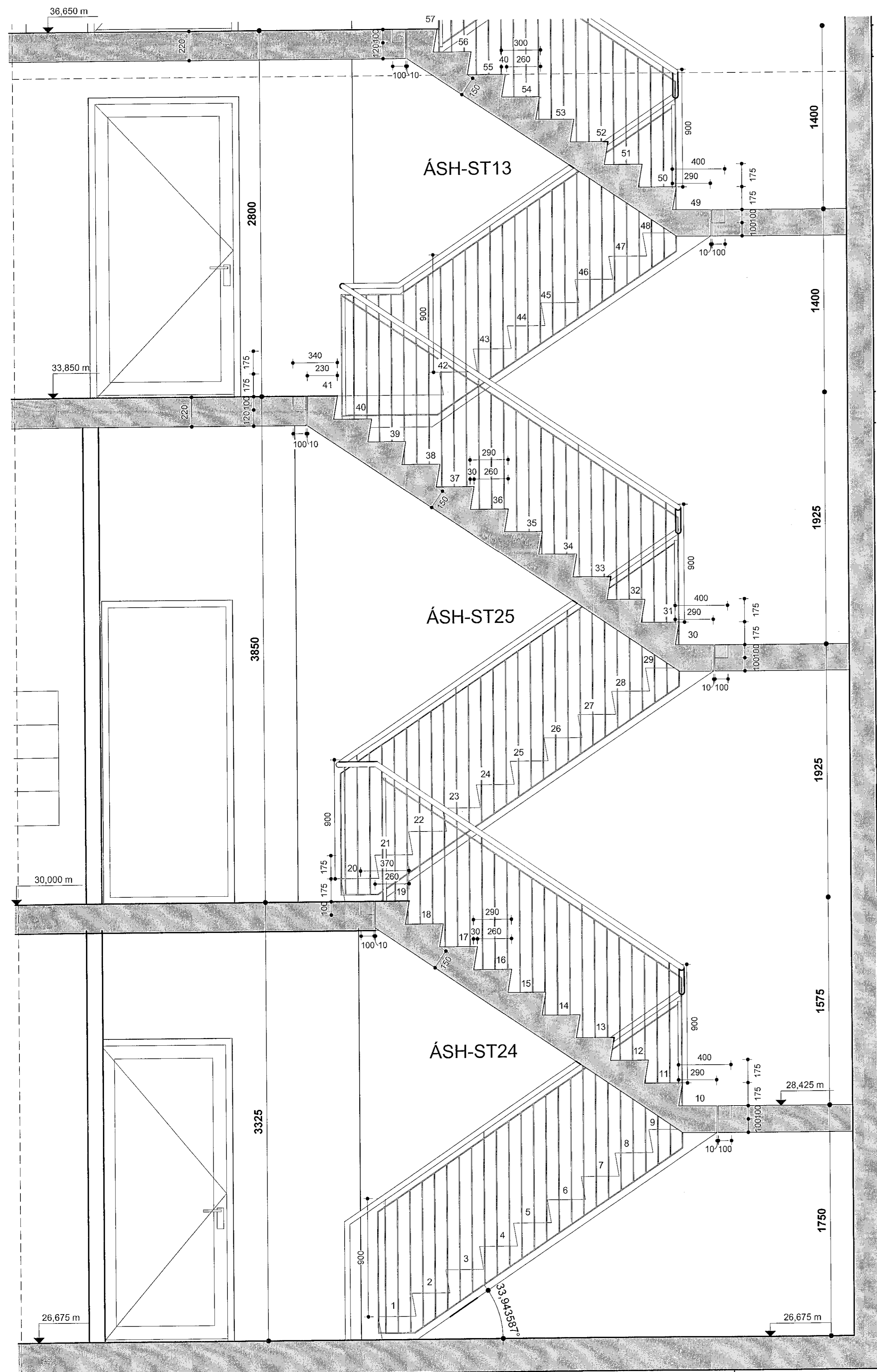
Stigi mhl.05 1/2 mkv: 1 : 20
