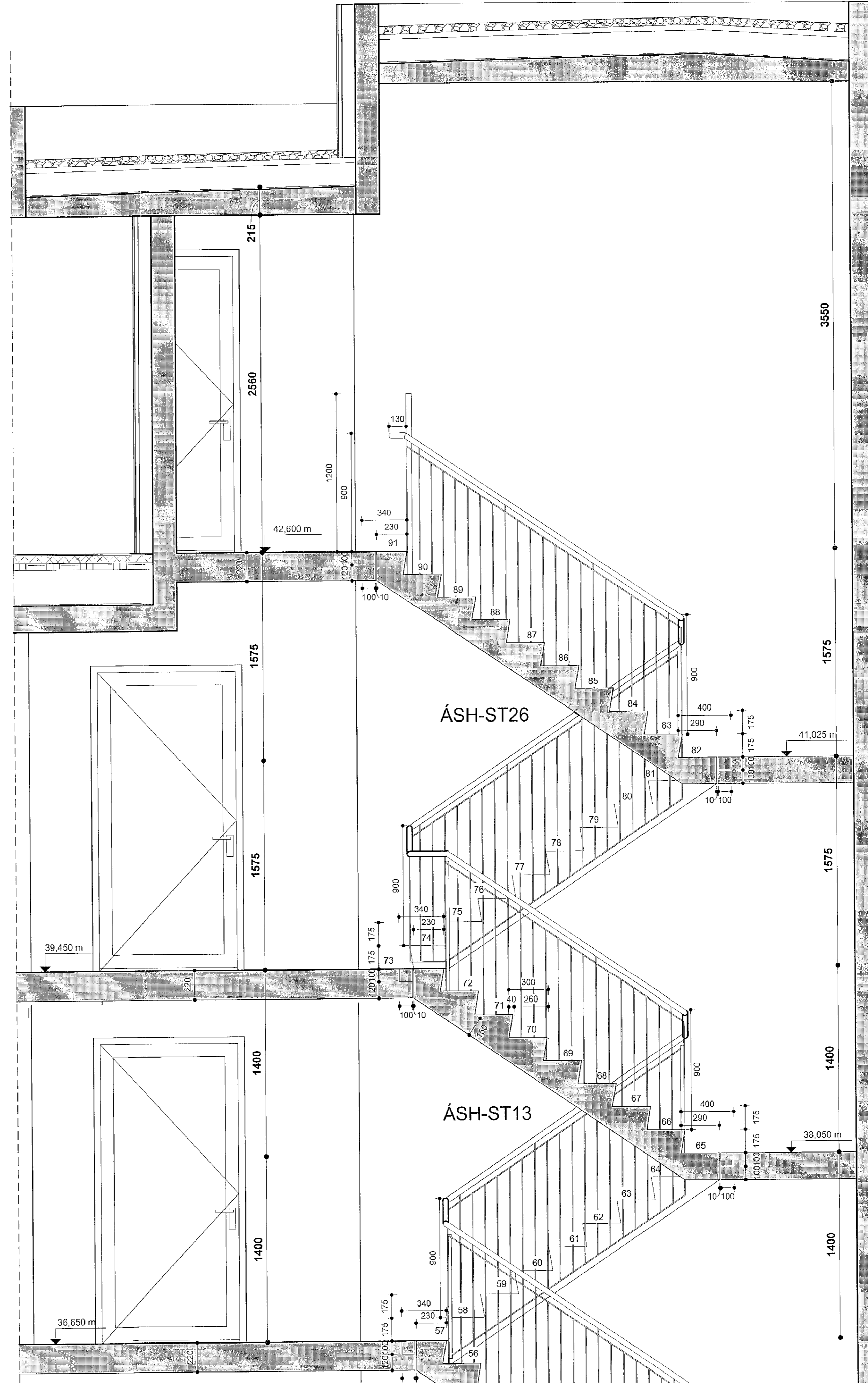
Stigi mhl.05 2/2 mkv: 1 : 20
