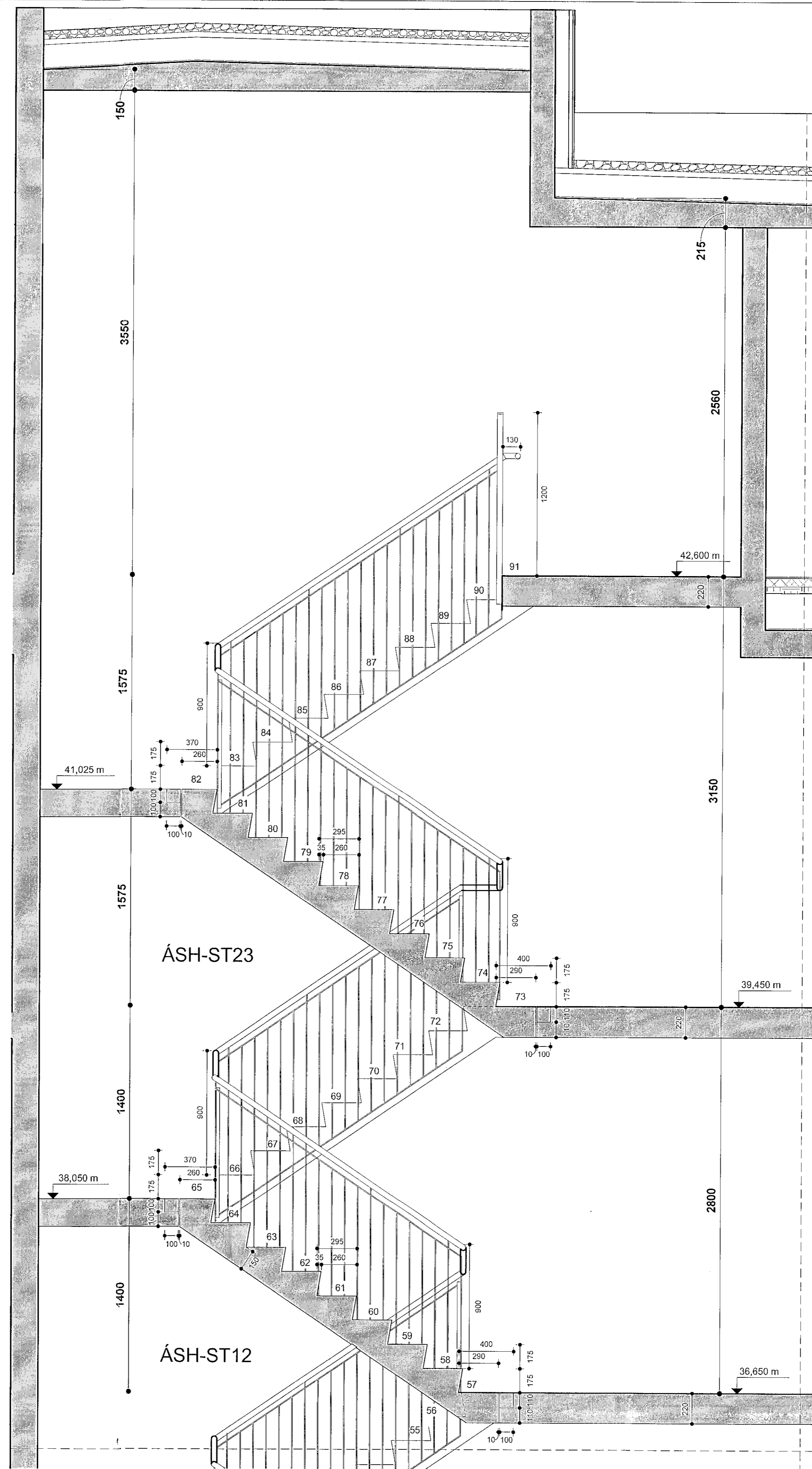
Stigi 2 mhl.05 2/2 mkv: 1 : 20
