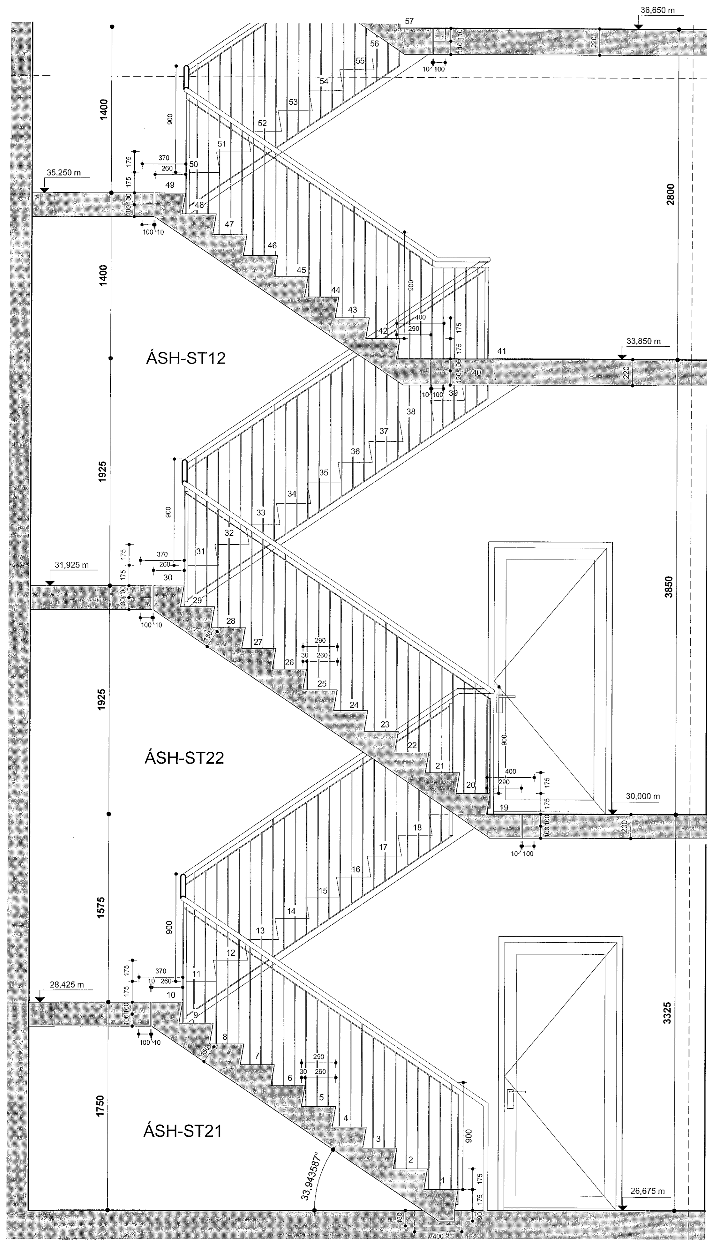
Stigi 2 mhl.05 1/2 mkv: 1 : 20
