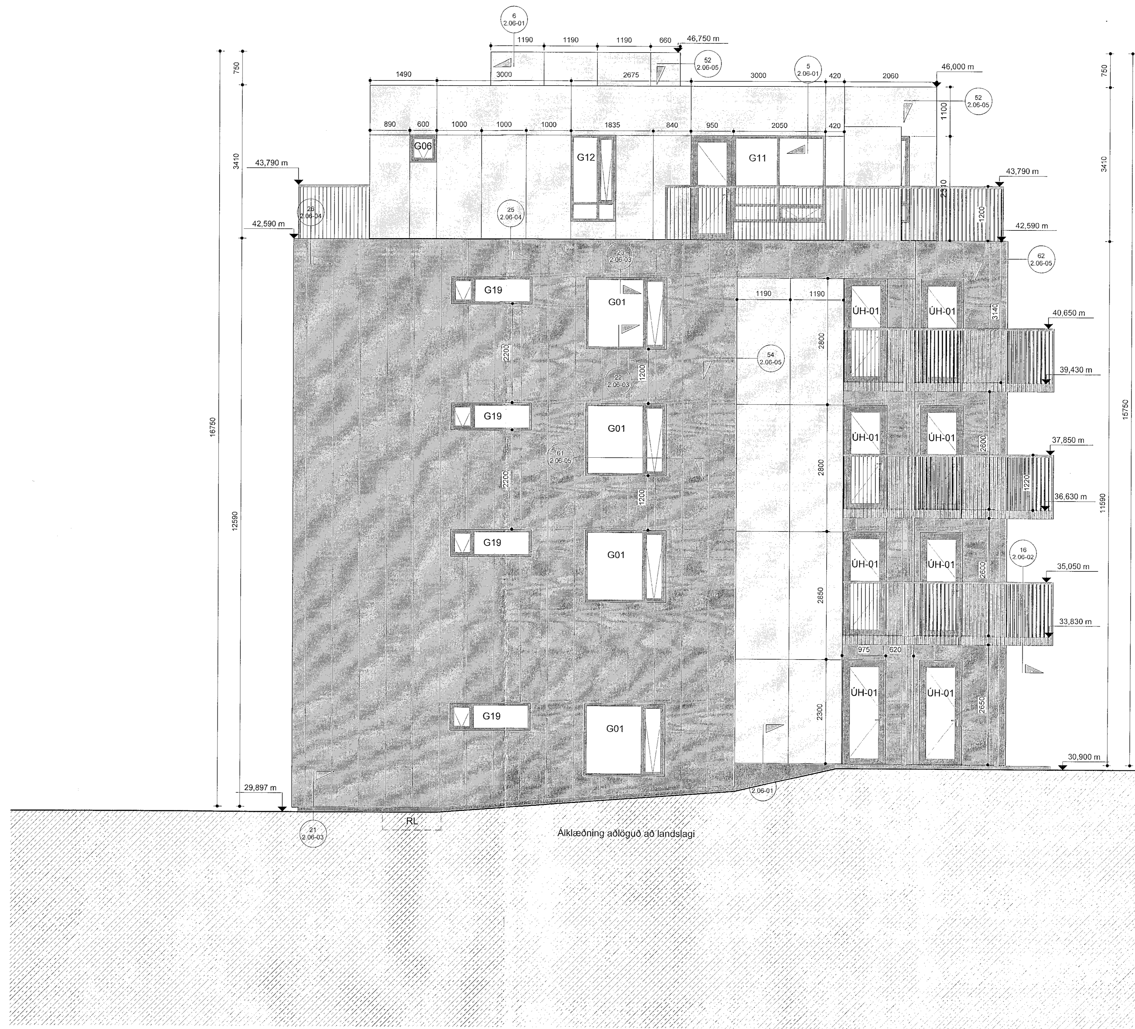
Áshamar 24 ásýnd norður verkt. mkv. 1 : 50
