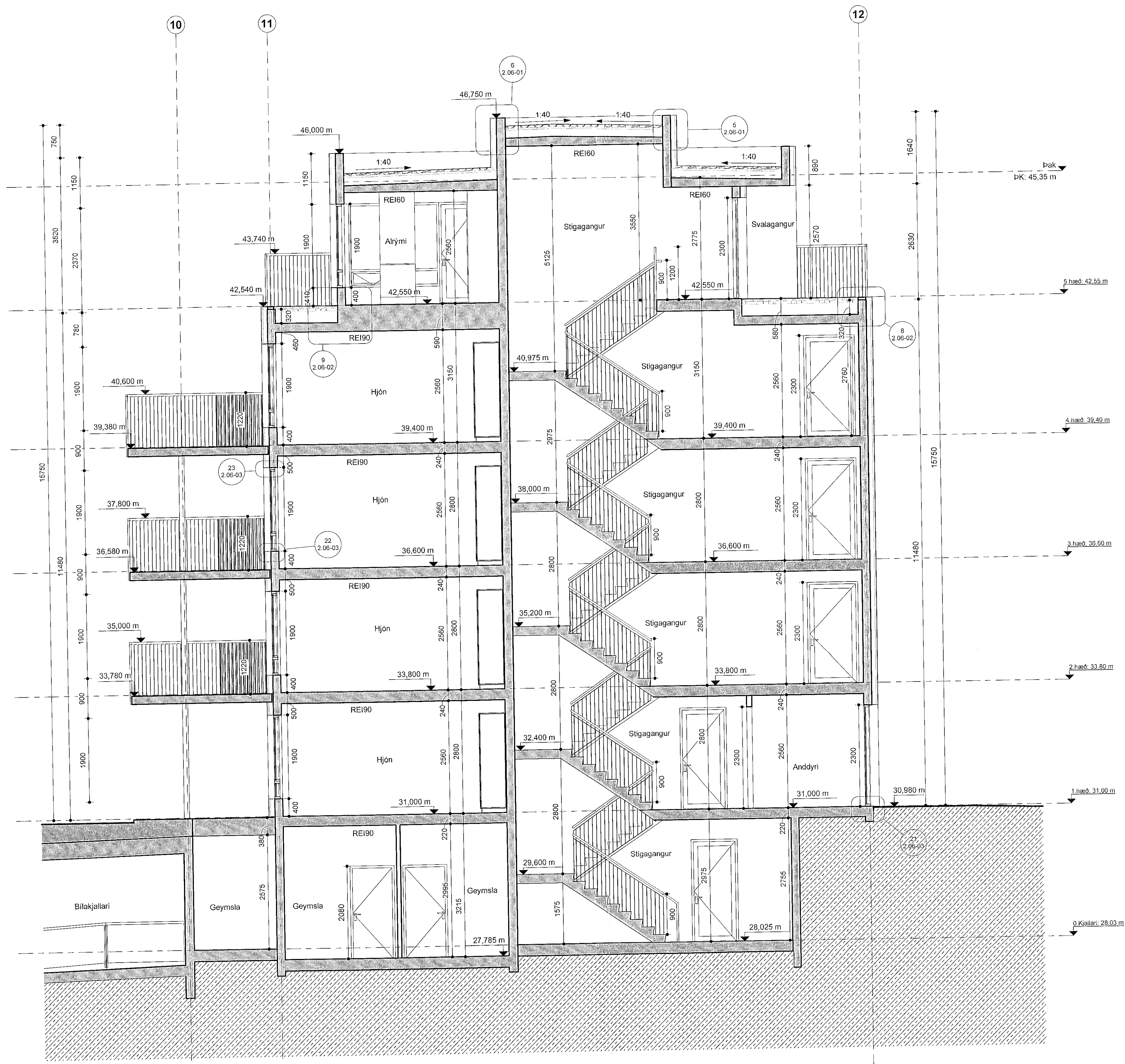
Áshamar 26 mhl.06 - snið - j-j mkv: 1 : 50
