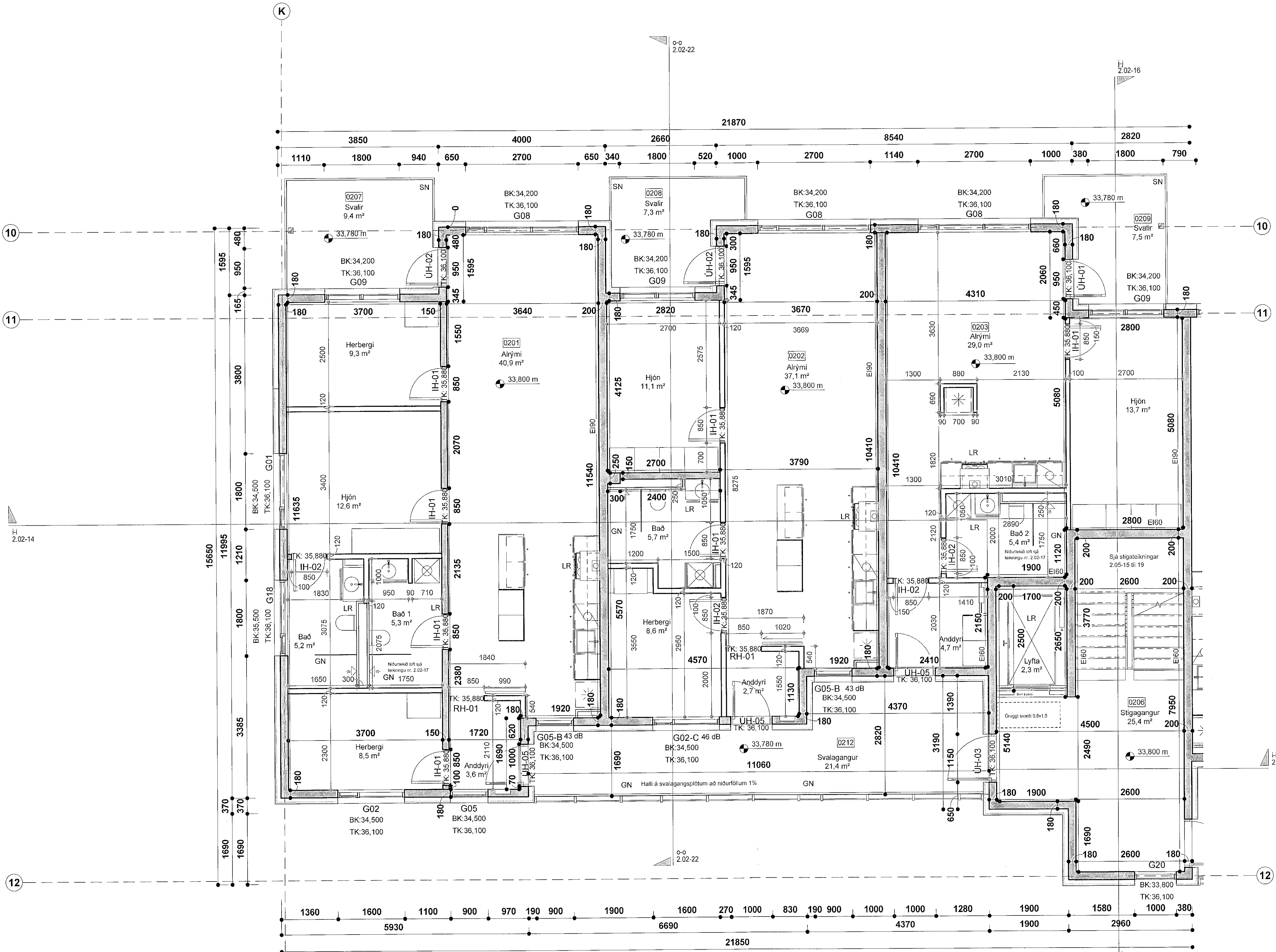
Áshamar 26 - 2.hæð - hluti 1 mkv: 1 : 50
