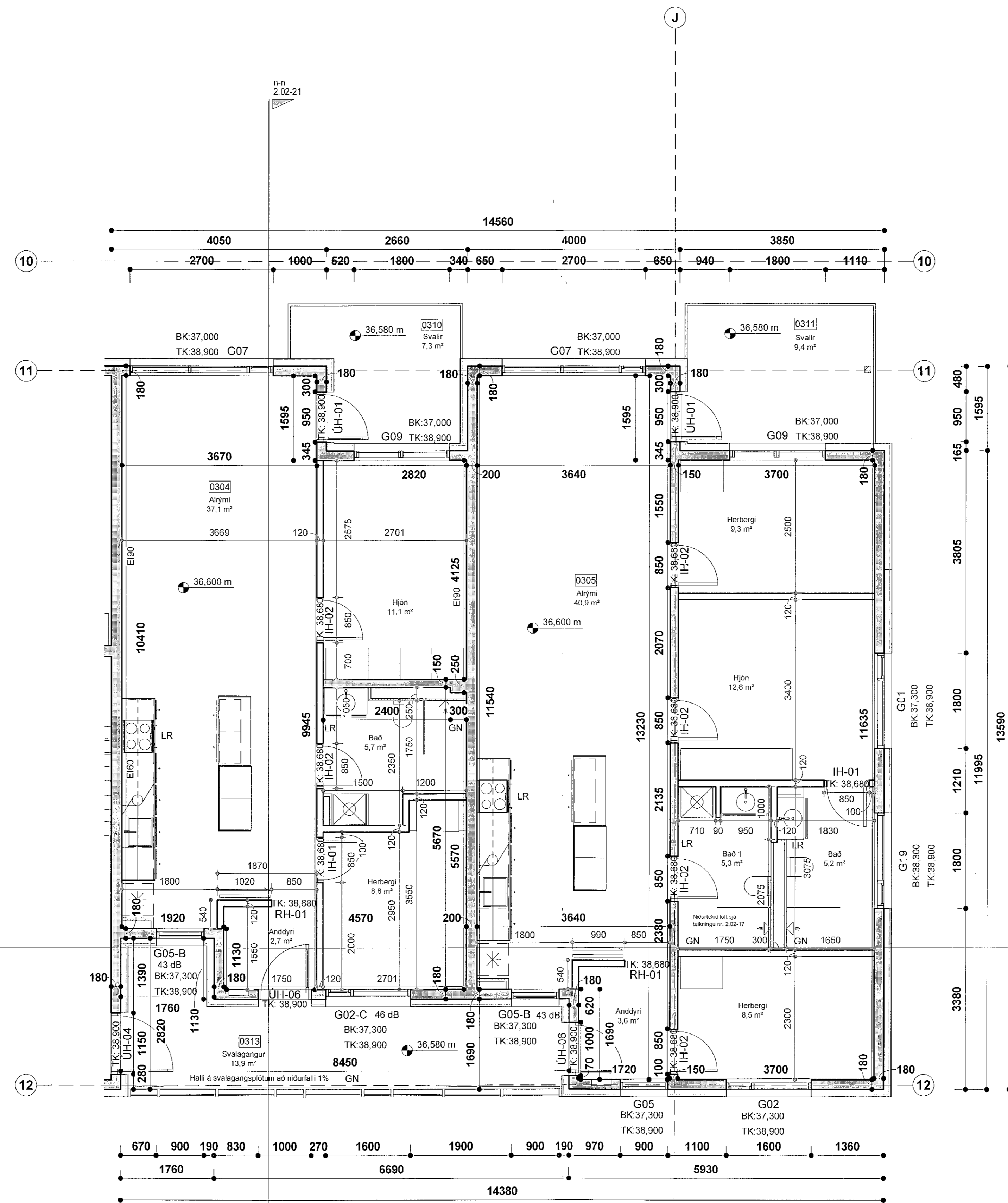
Áshamar 26 - 3.hæð - hluti 2 mkv: 1 : 50
