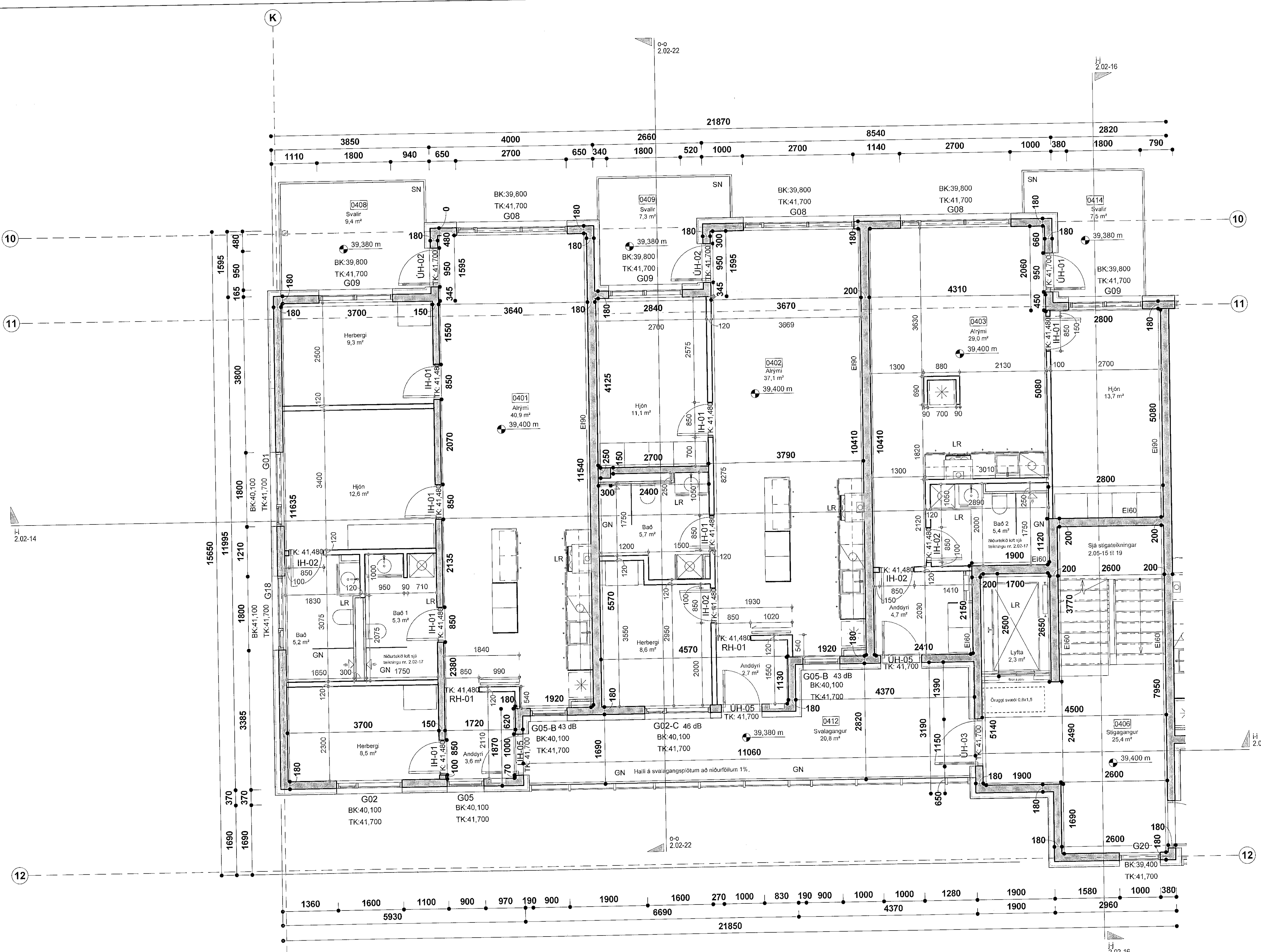
Áshamar 26 - 4. hæð - hluti 1 mkv: 1 : 50
