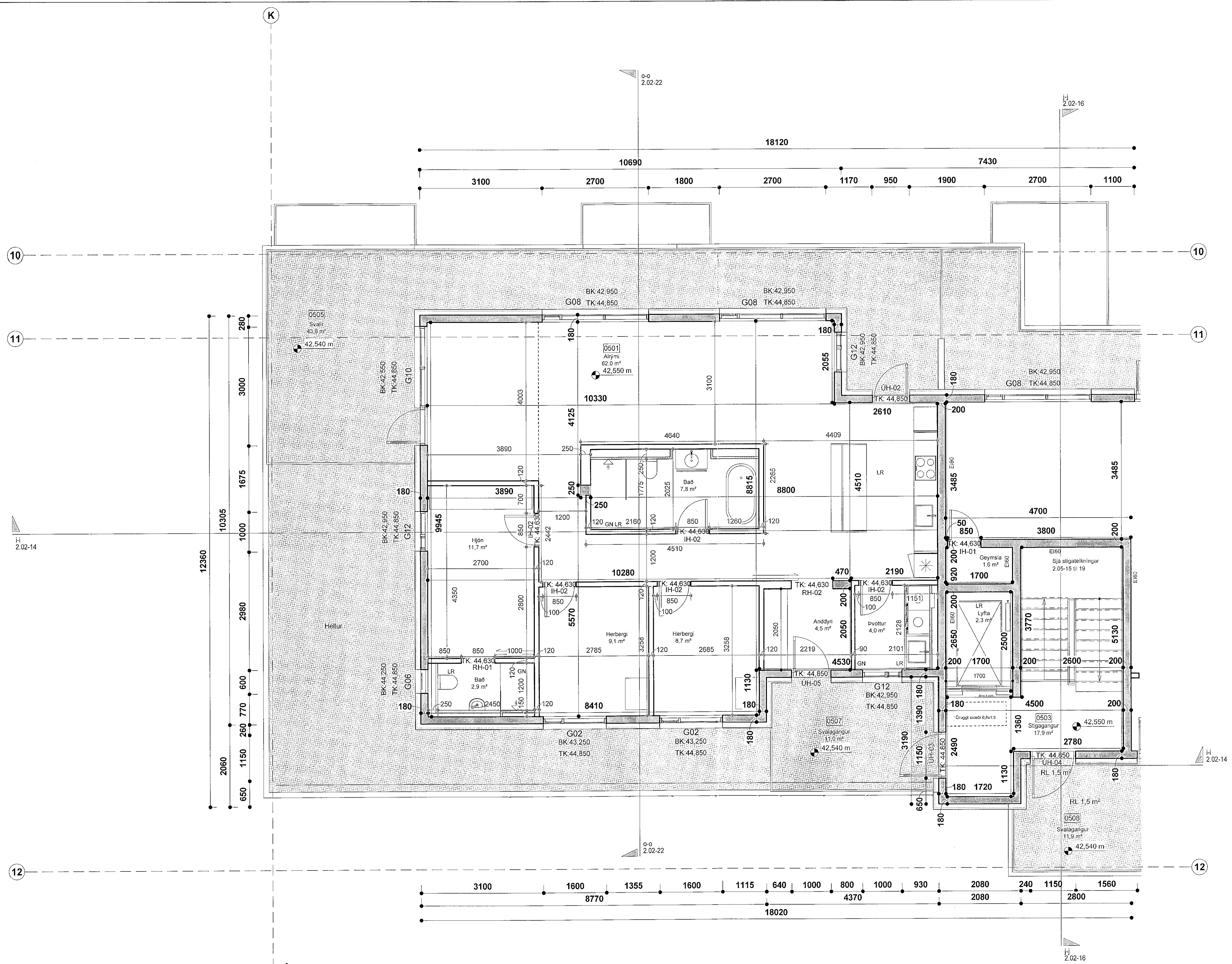
Ashamar 26 - 5.hæð - hluti 1 mkv: 1 : 50
