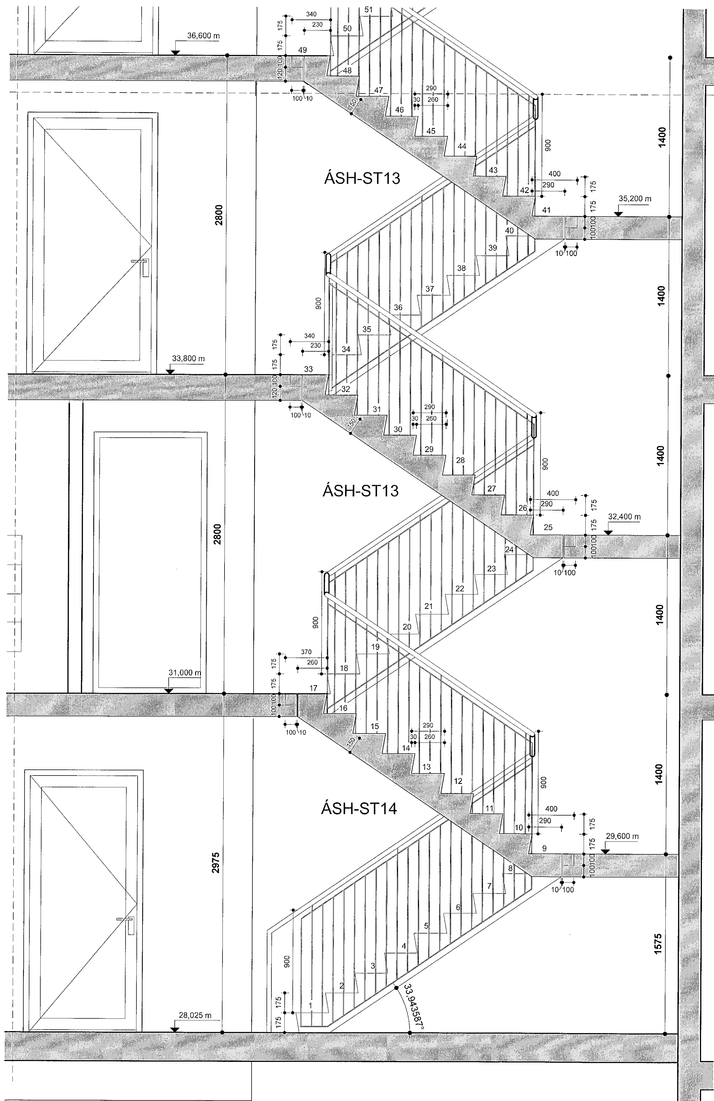
Stigi 8 mhl.06 1/2 mkv: 1 : 20
