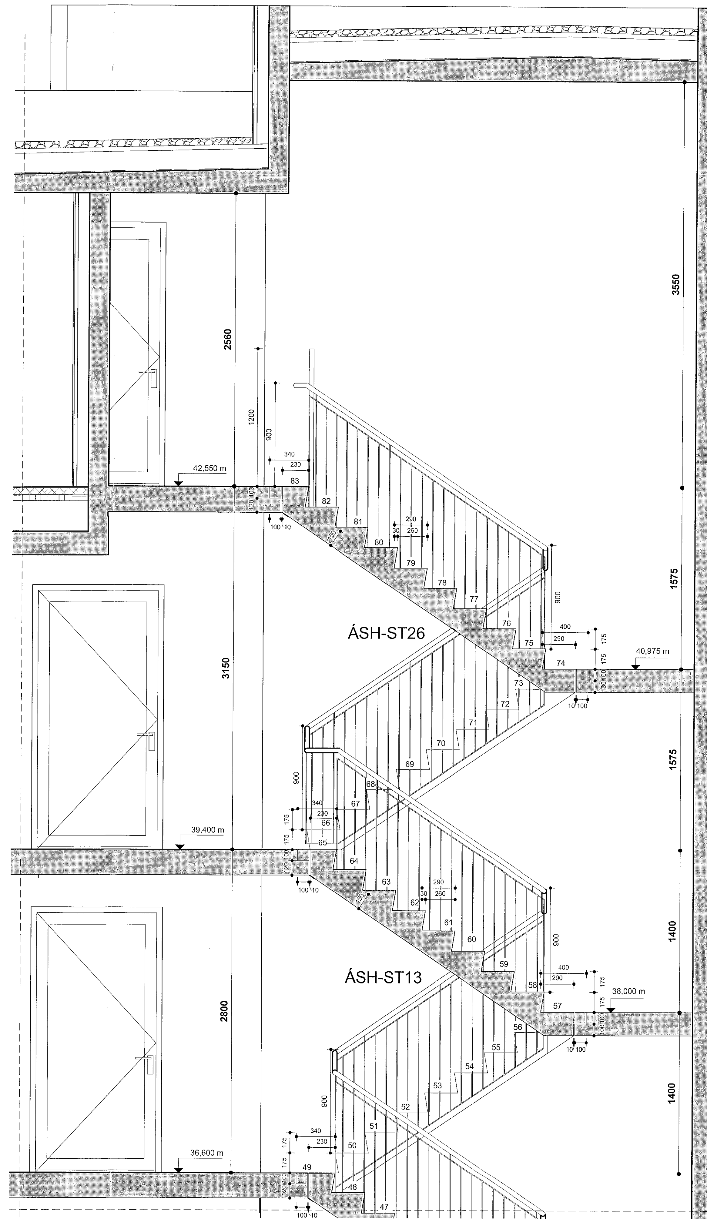
Stigi 8 mhl.06 2/2 mkv: 1 : 20
