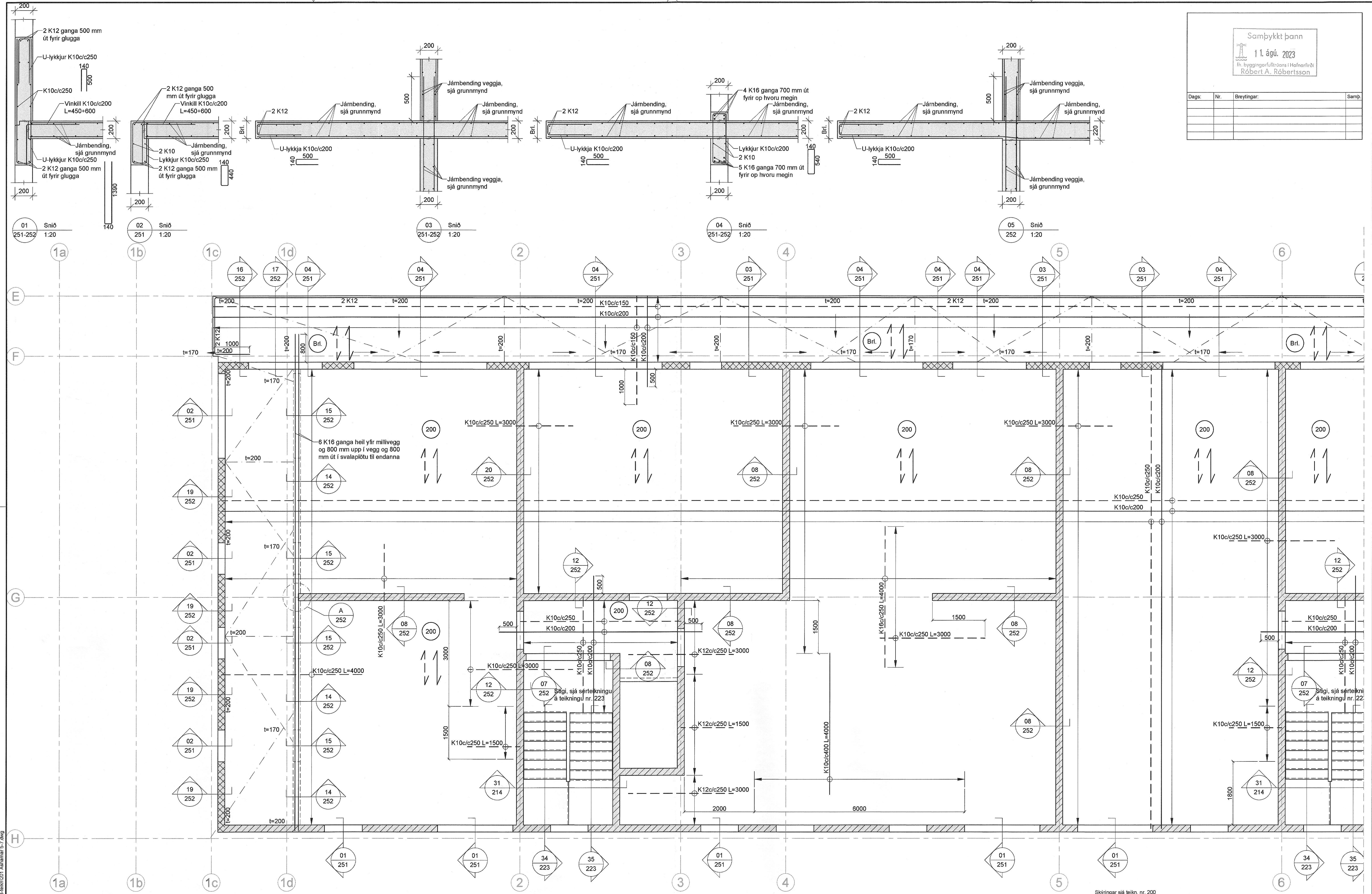
Grunnmynd 5. hæðar, 1:50
