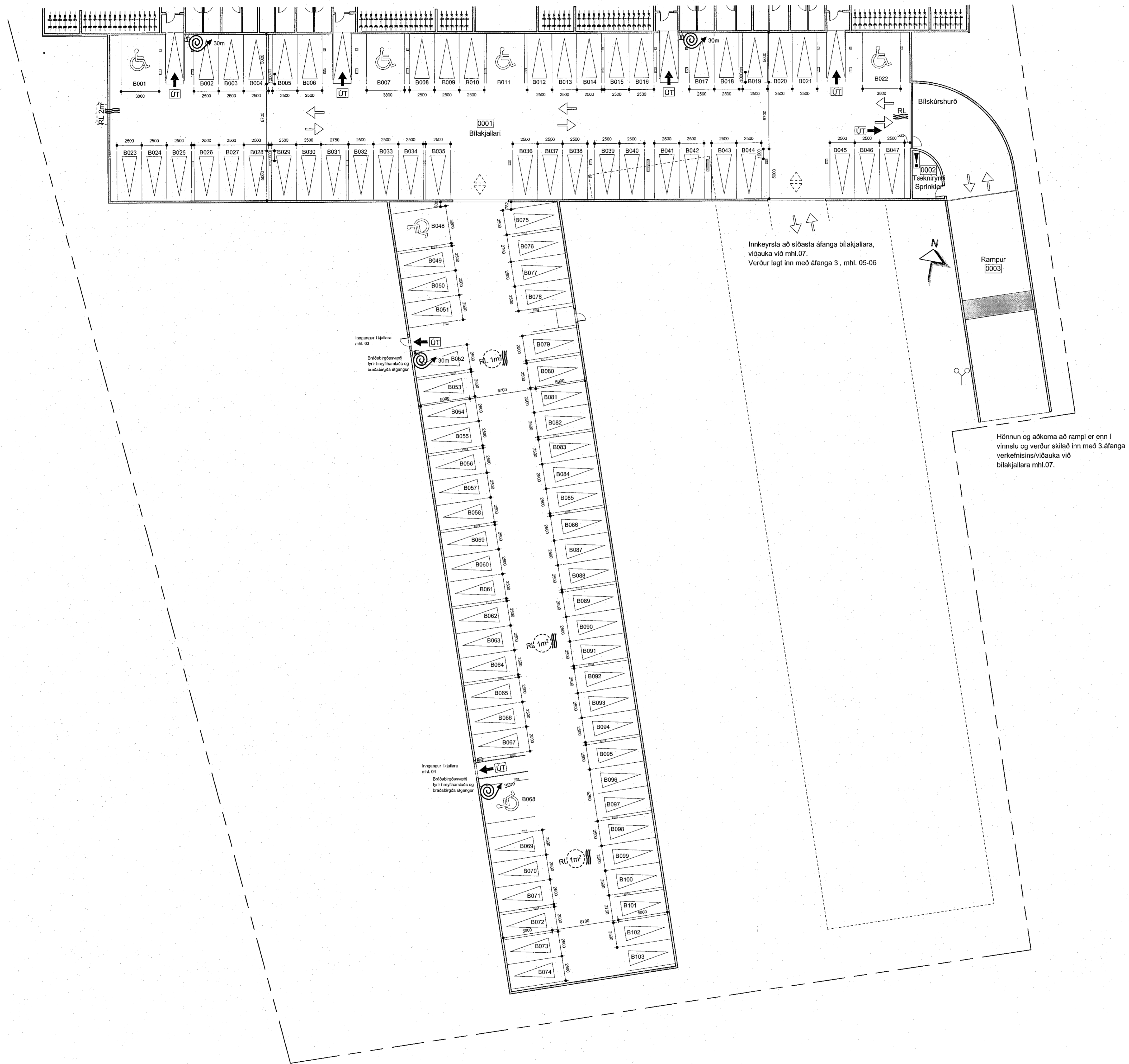
-1. Bilakjallari Yfirlit - mhl. 07 mkv: 1 : 200
