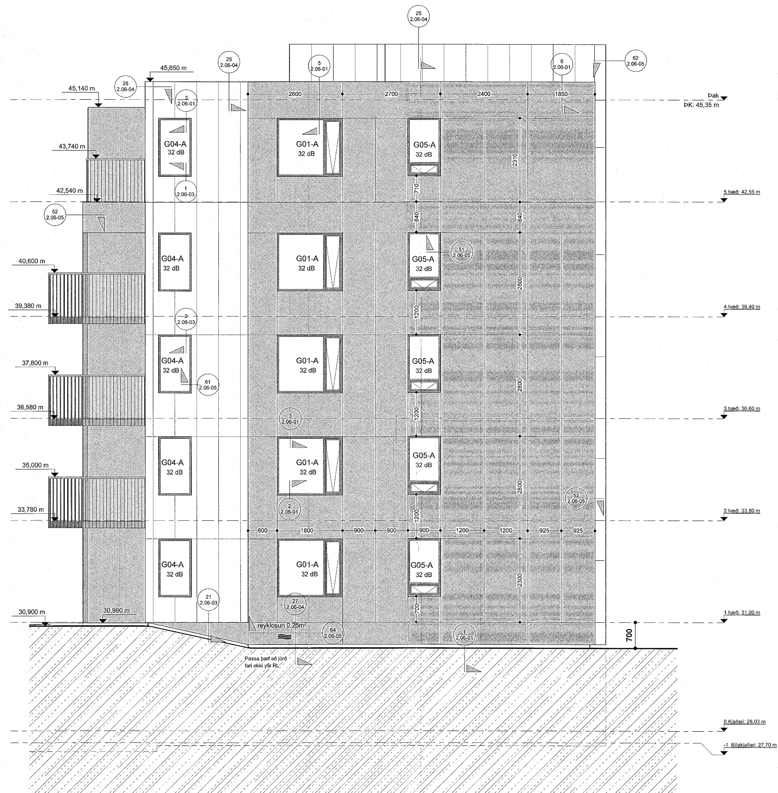
Áshamar 12-14, mhl.01-02 ásýnd austur verkt. mkv: 1 : 50
