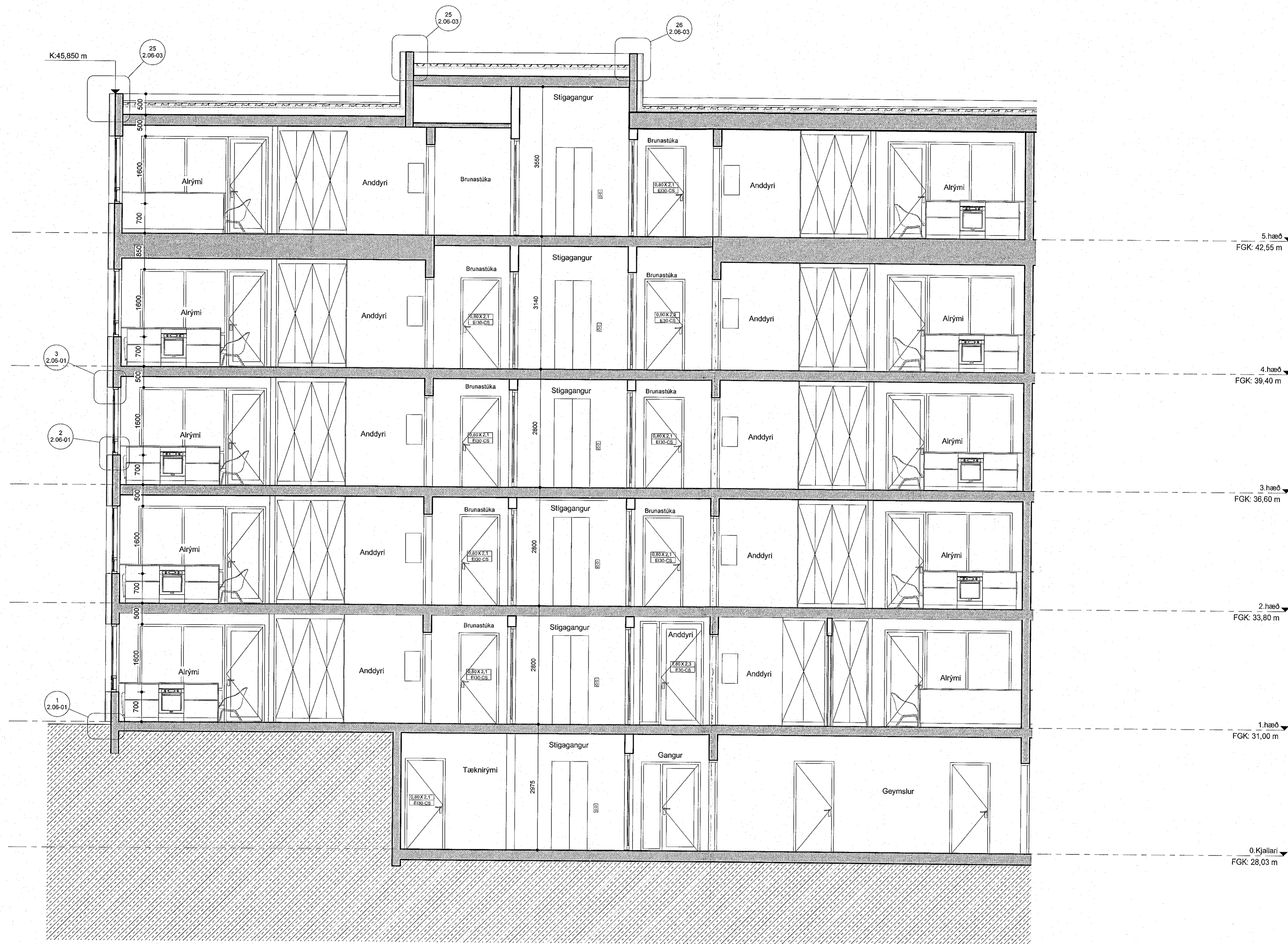
Áshamar 12-18 mhl.01-02 - snið a-a - hluti 1 mkv: 1 : 50
