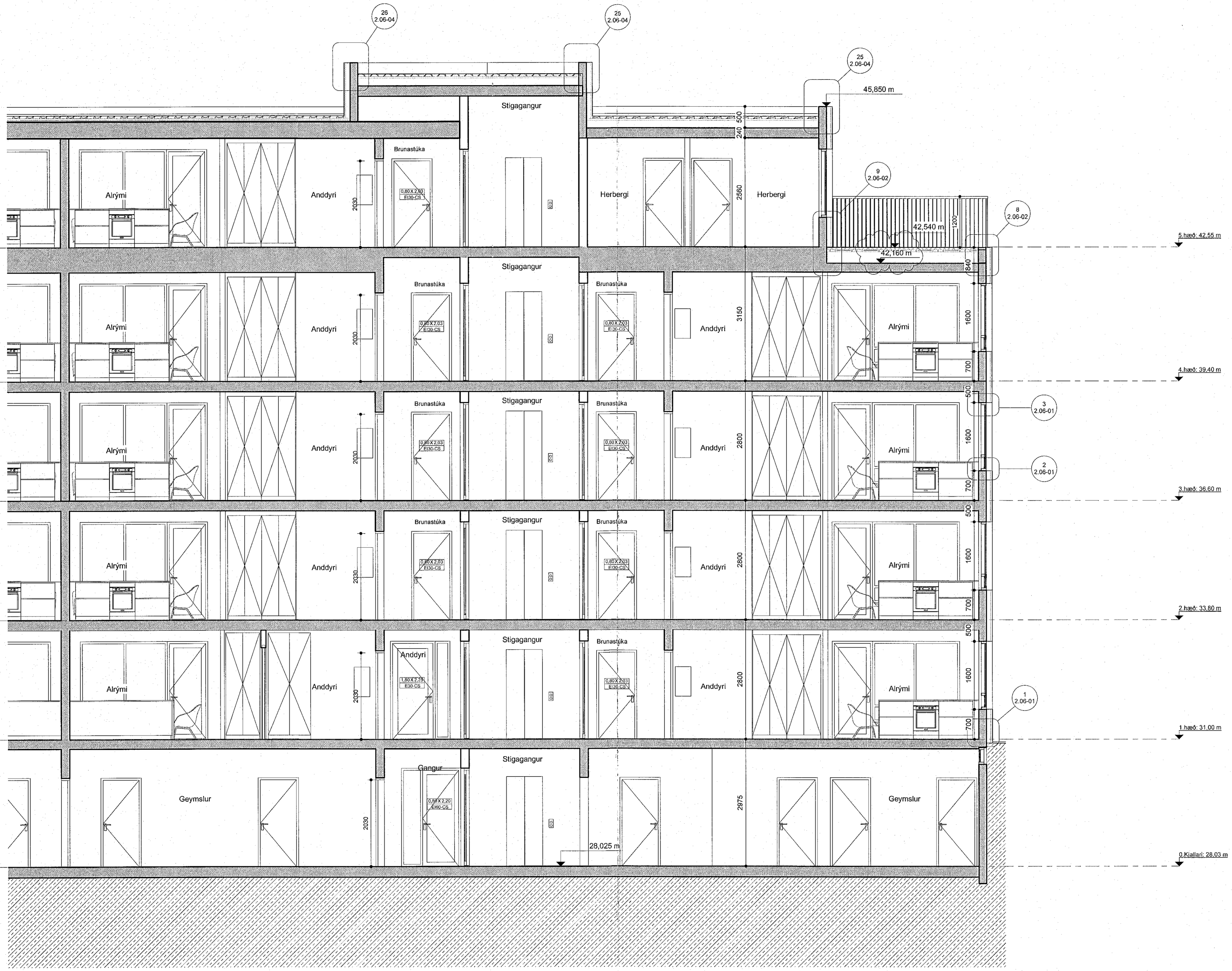
Áshamar 12-18 mhl.01-02 - snið a-a - hluti 2 mkv: 1 : 50
