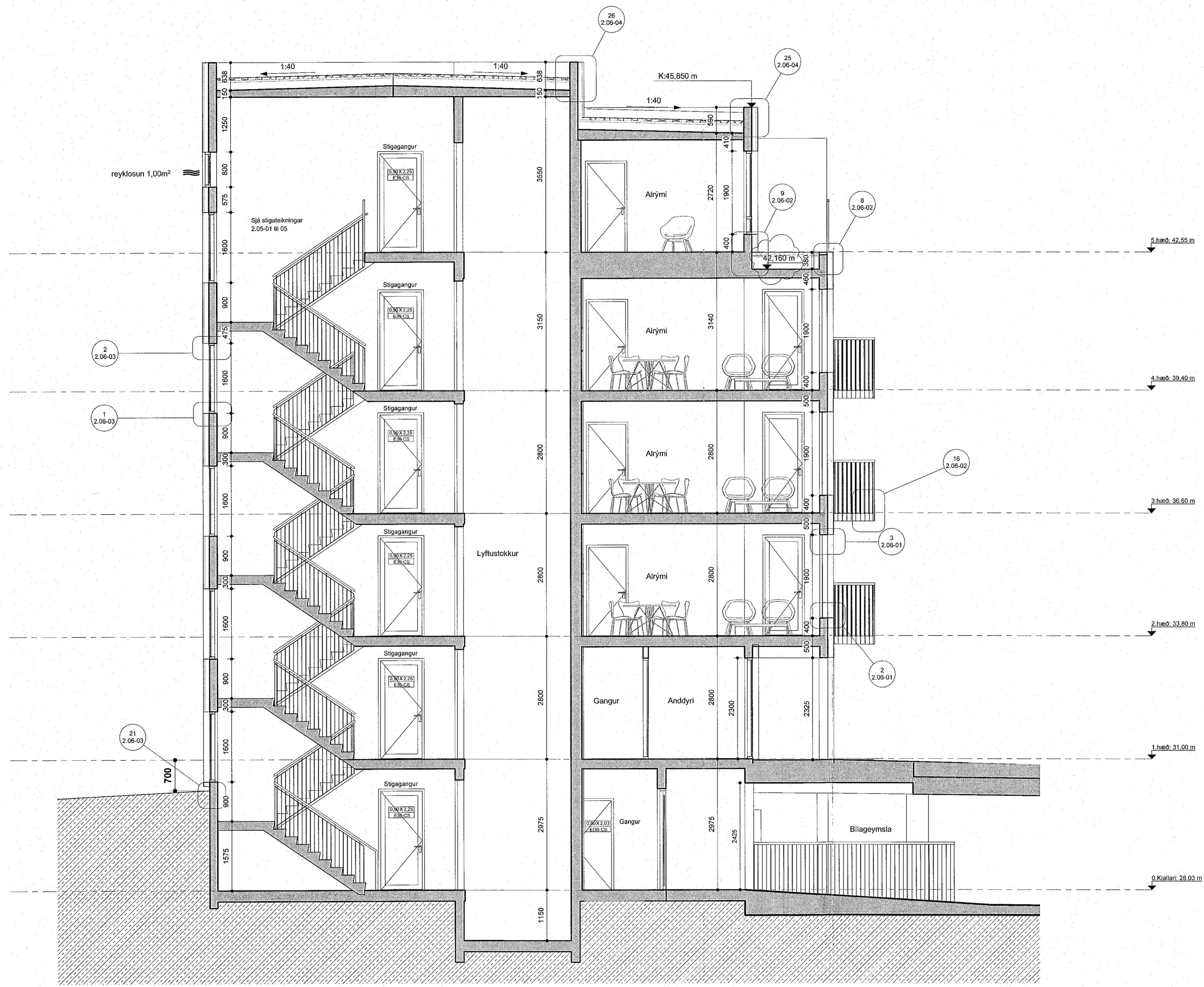
Áshamar 12-18 mhl.01 - snið b-b mkv. 1 : 50
