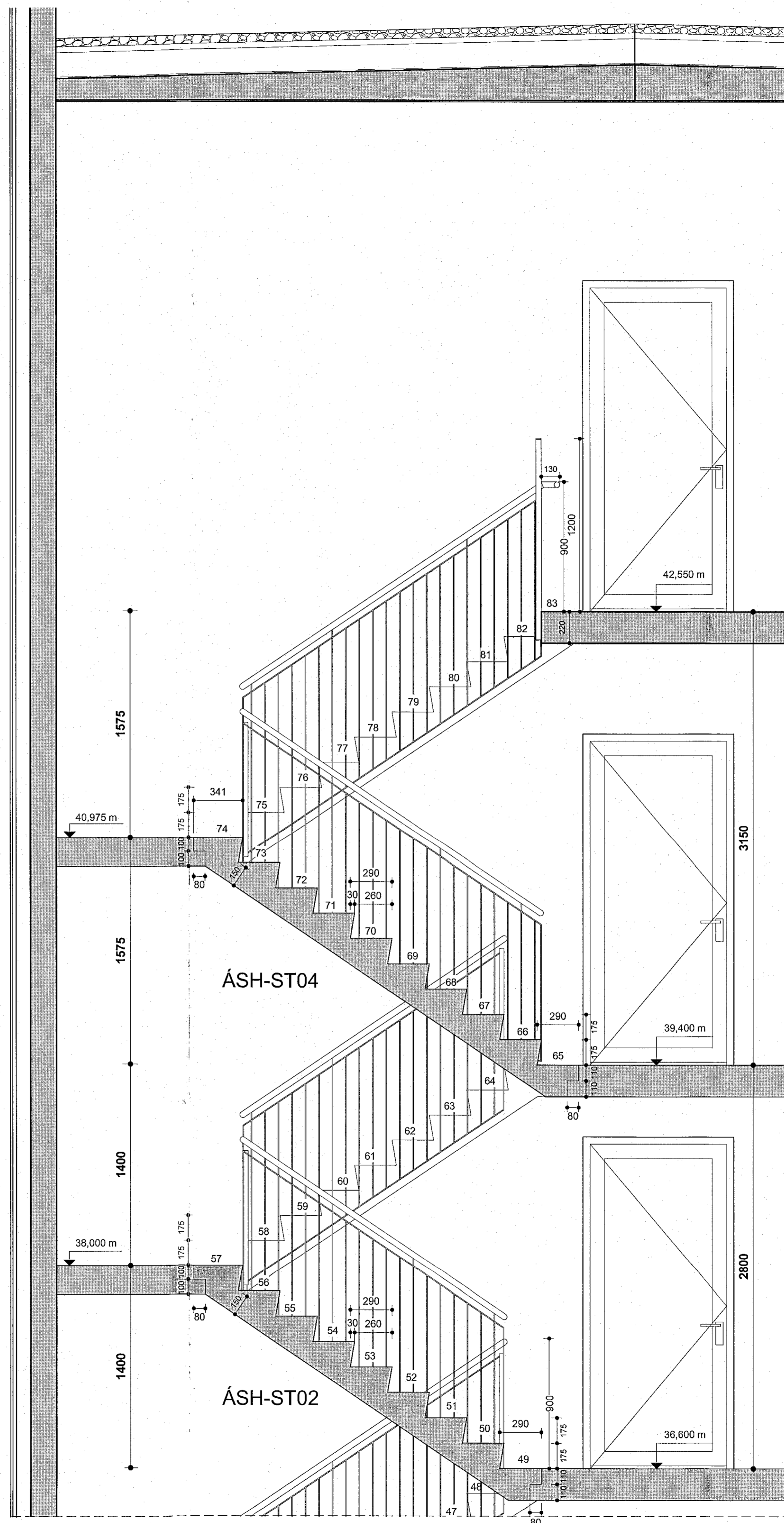
Snið stigi 1 - 2/2 mhl.01-02 mkv: 1 : 20
