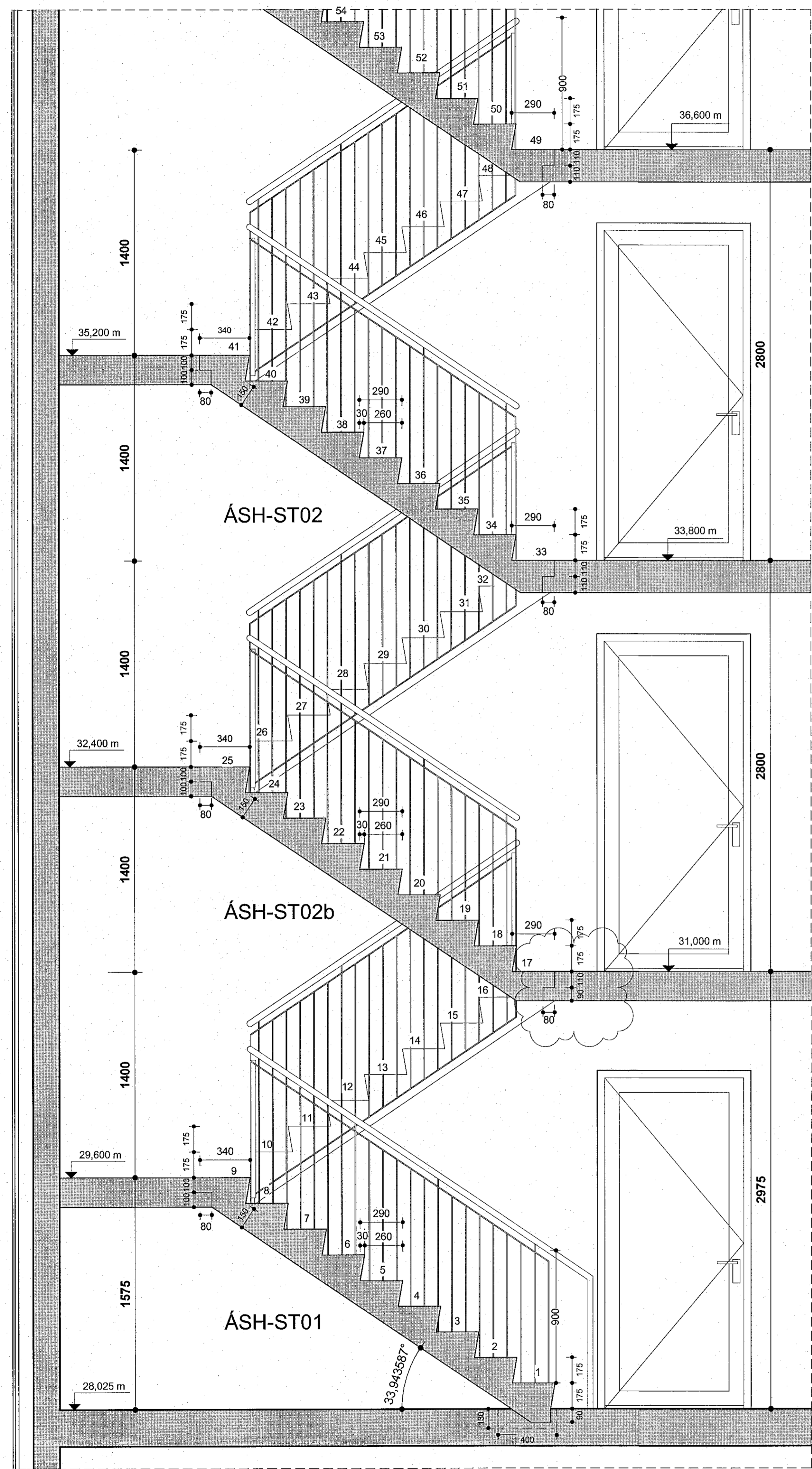
Snið stigi 1 - 1/2 mhl.01-02 mkv: 1 : 20
