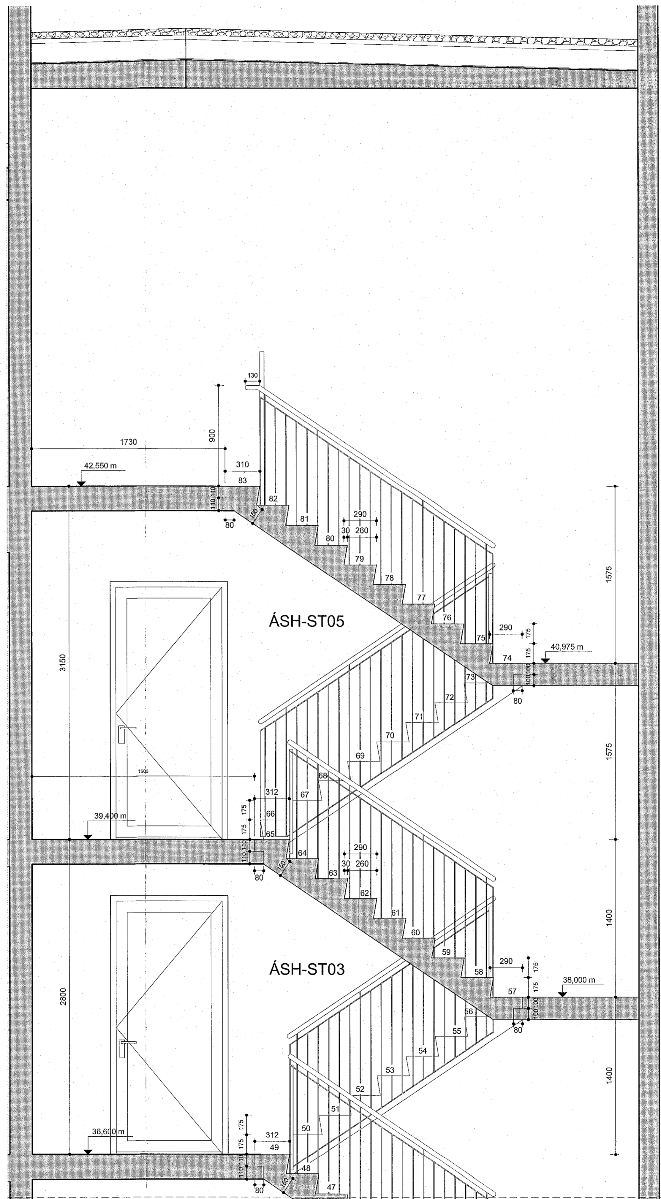
Snið stigi 2 - 2/2 mhl.01-02 mkv: 1 : 20
