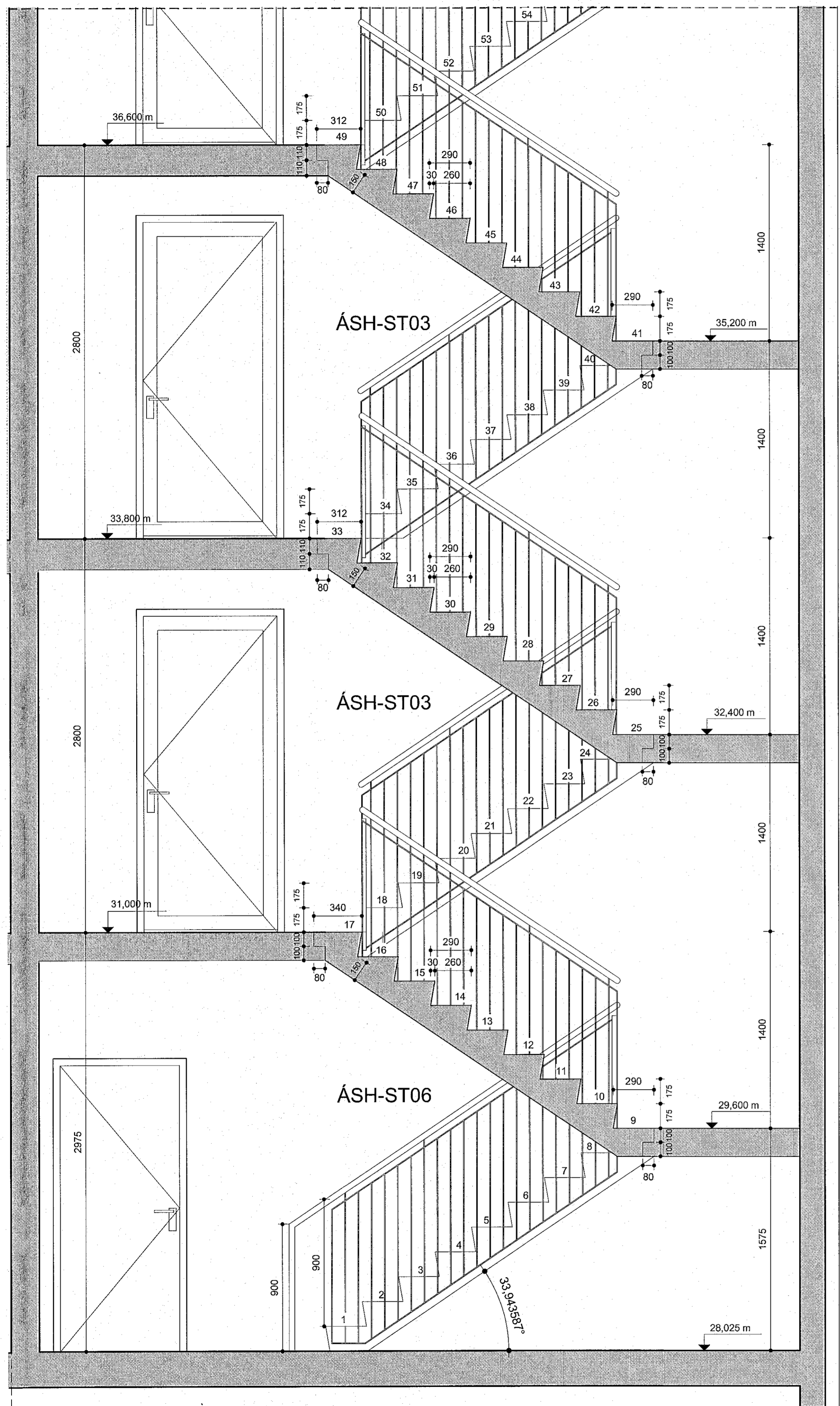
Snið stigi 2 - 1/2 mhl.01-02 mkv: 1 : 20
