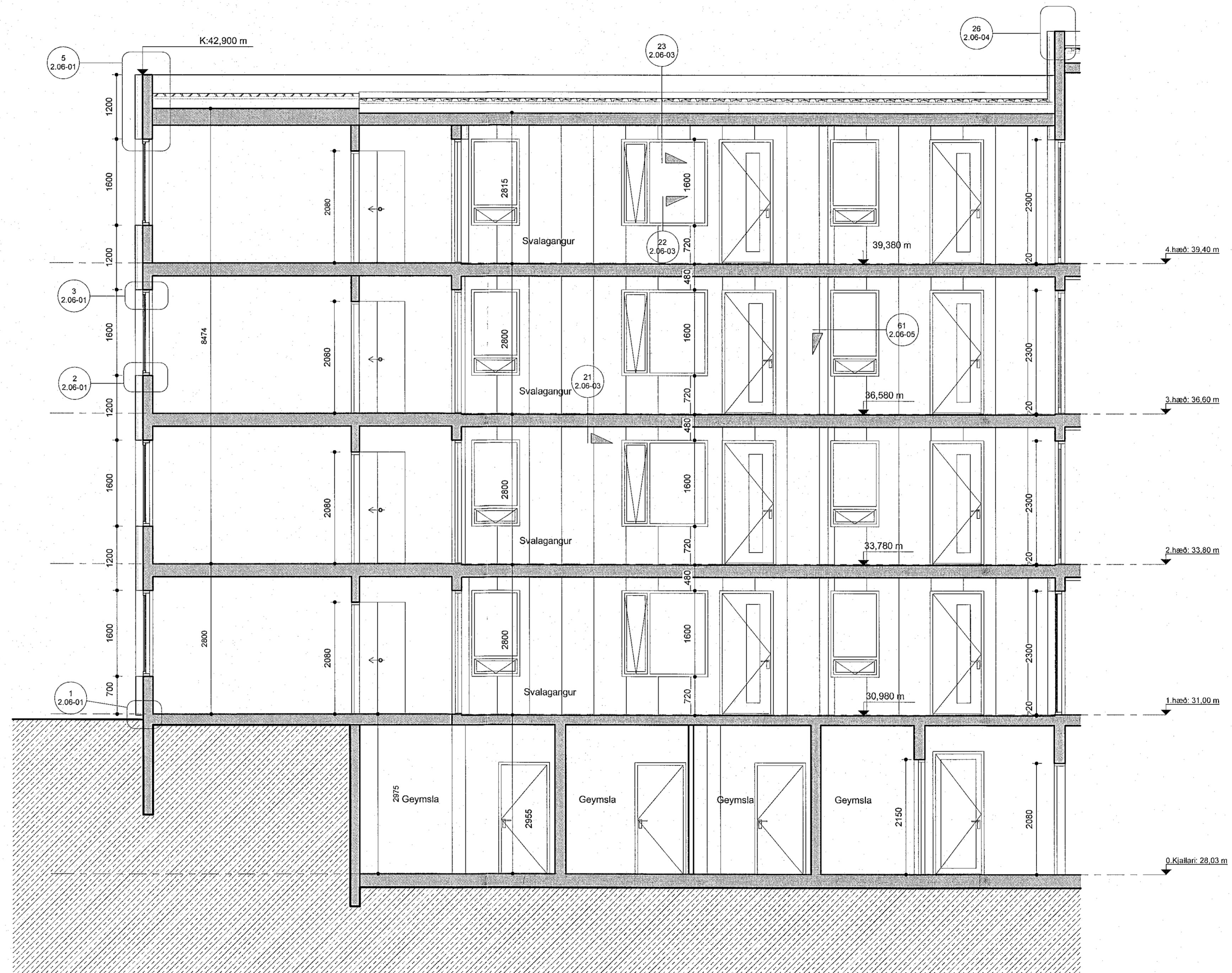
Áshamar 20-22 mhl.03-04 - snið d-d - hluti 1 mkv: 1 : 50
