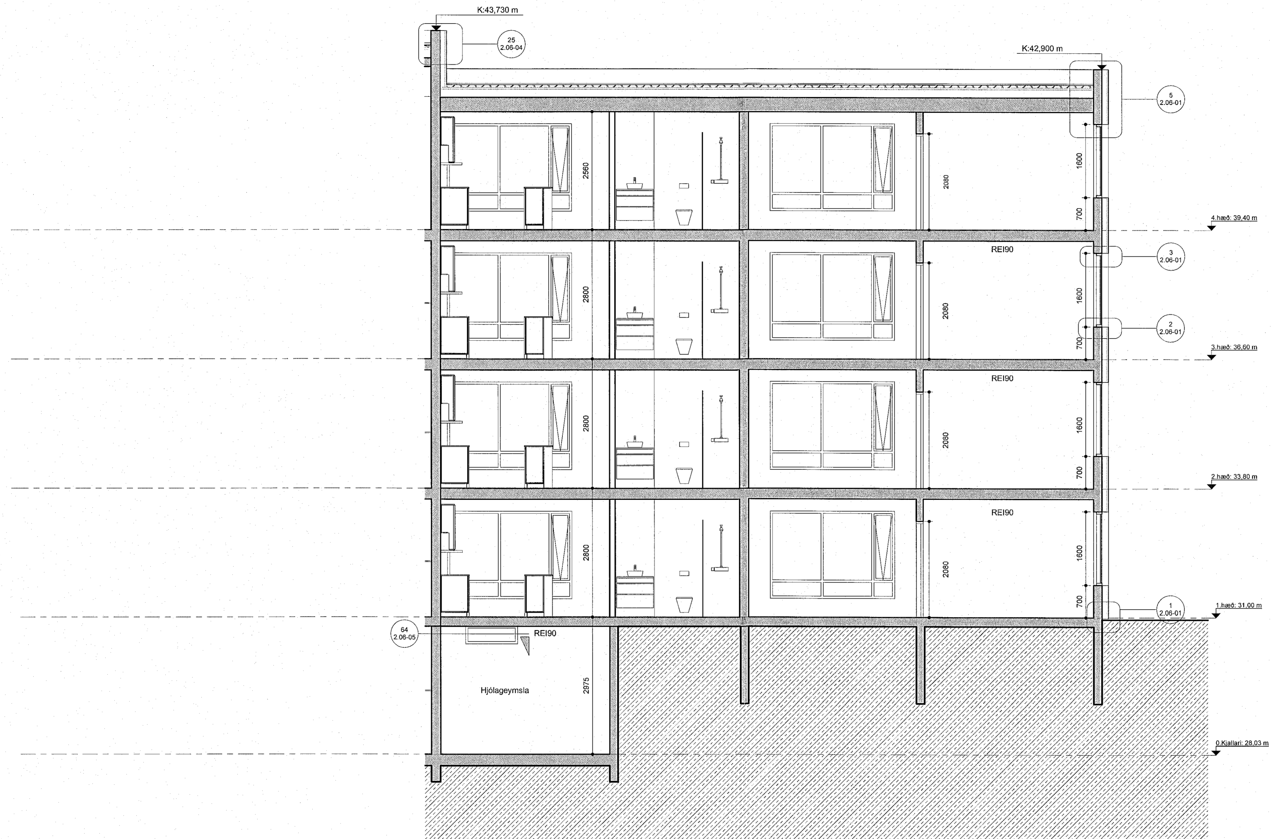
Áshamar 20-22 mhl.03-04 - snið d-d - hluti 2 mkv: 1 : 50
