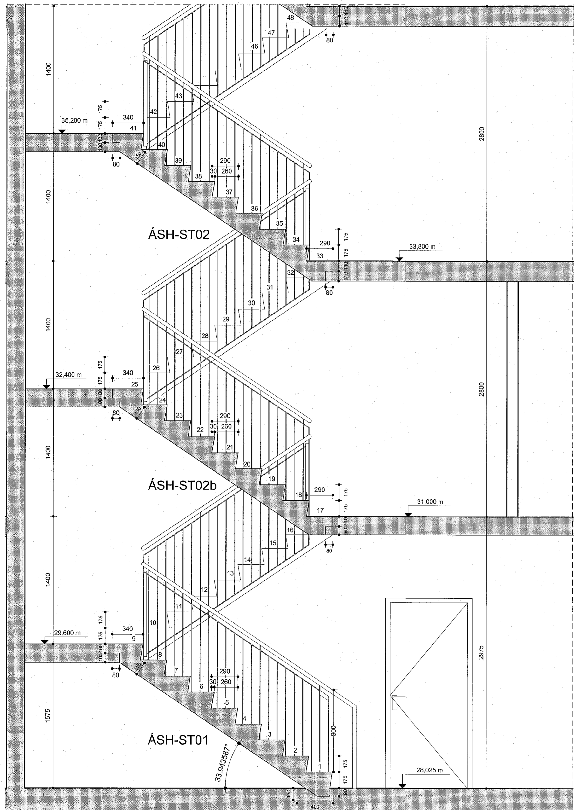
Stigi 3 - 1/2 mhl.03-04 mkv: 1 : 20
