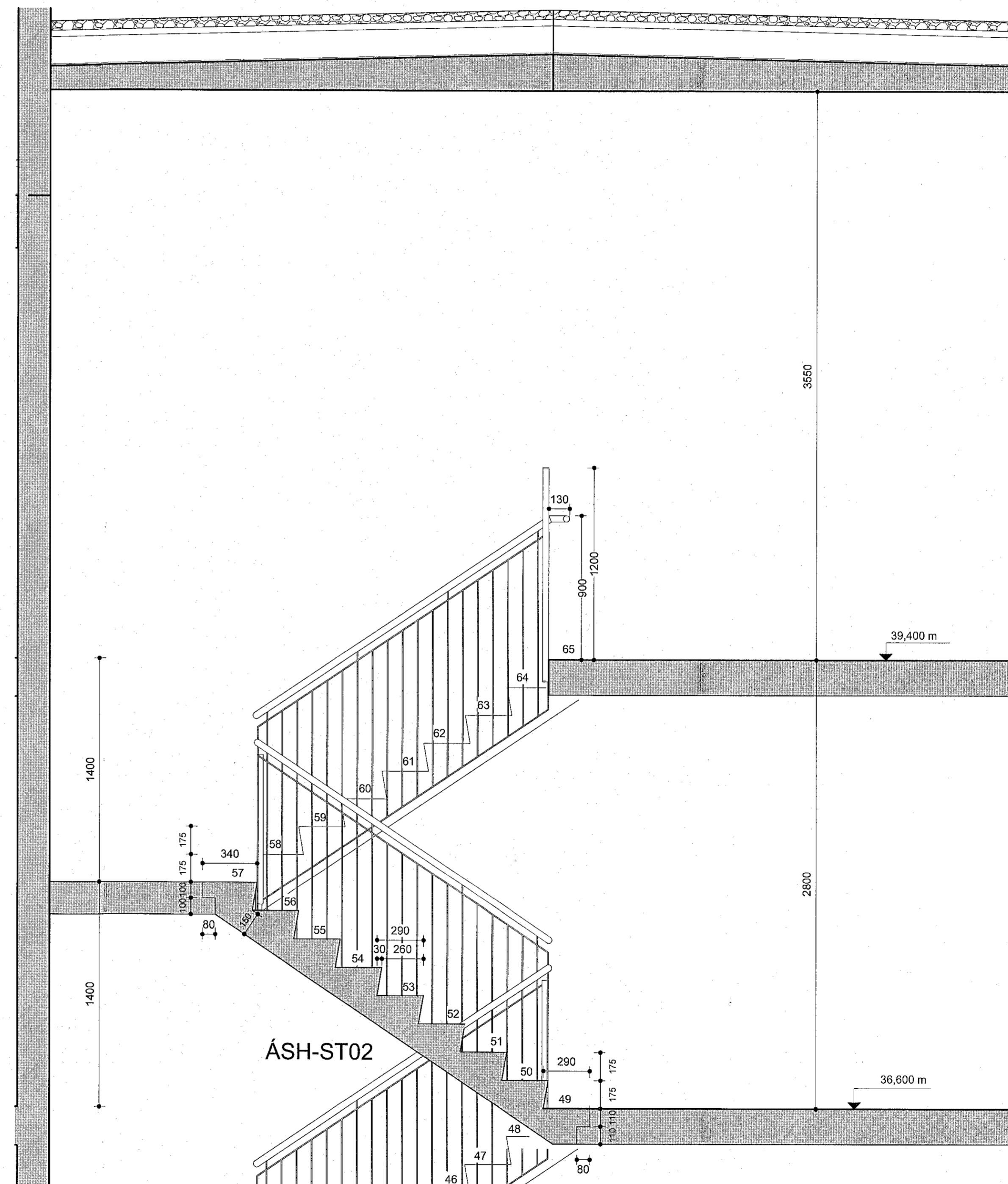
Stigi 3 - 2/2 mhl.03-04 mkv: 1 : 20
