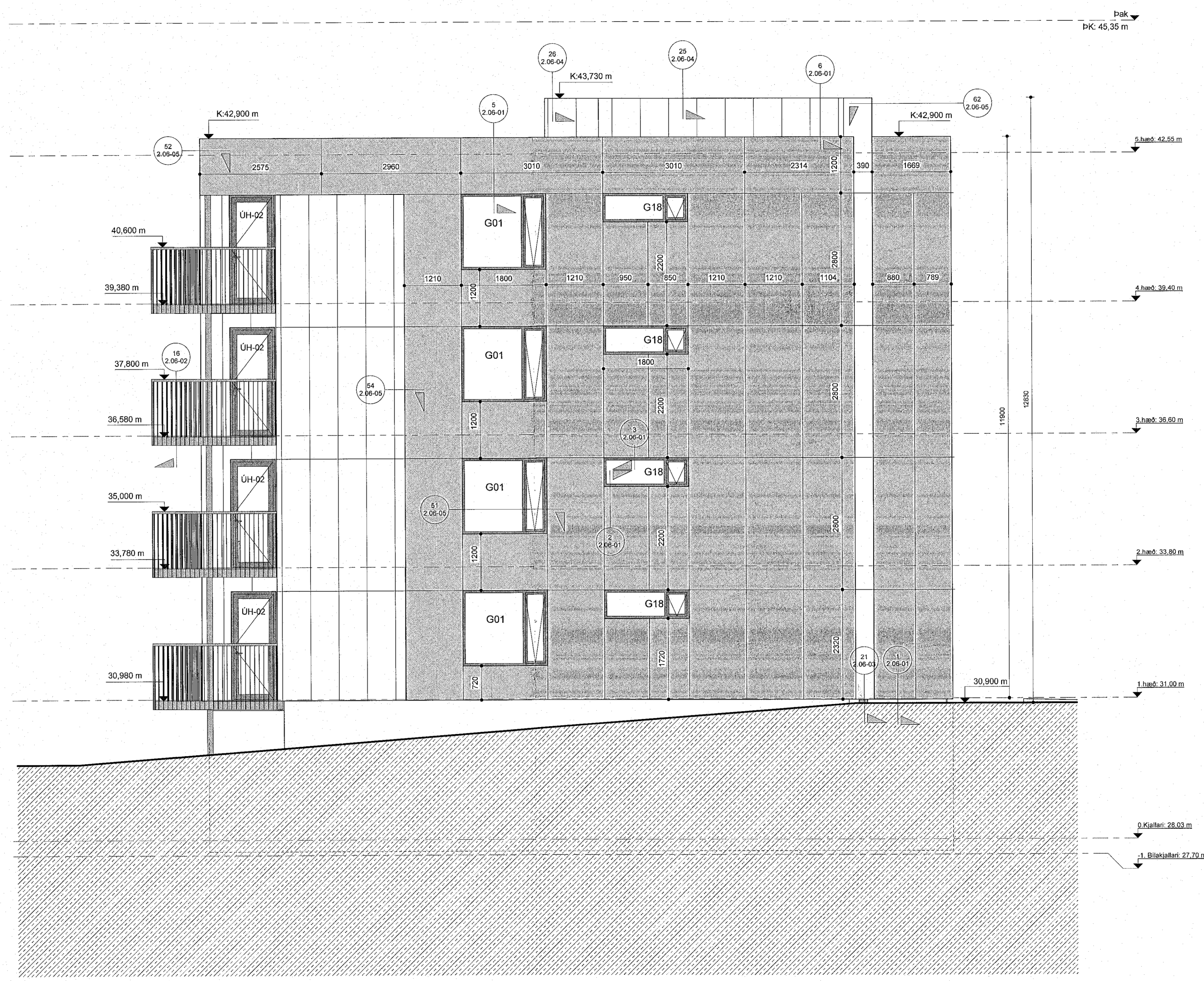
Áshamar 20 ásýnd suður verkt. mkv: 1 : 50
