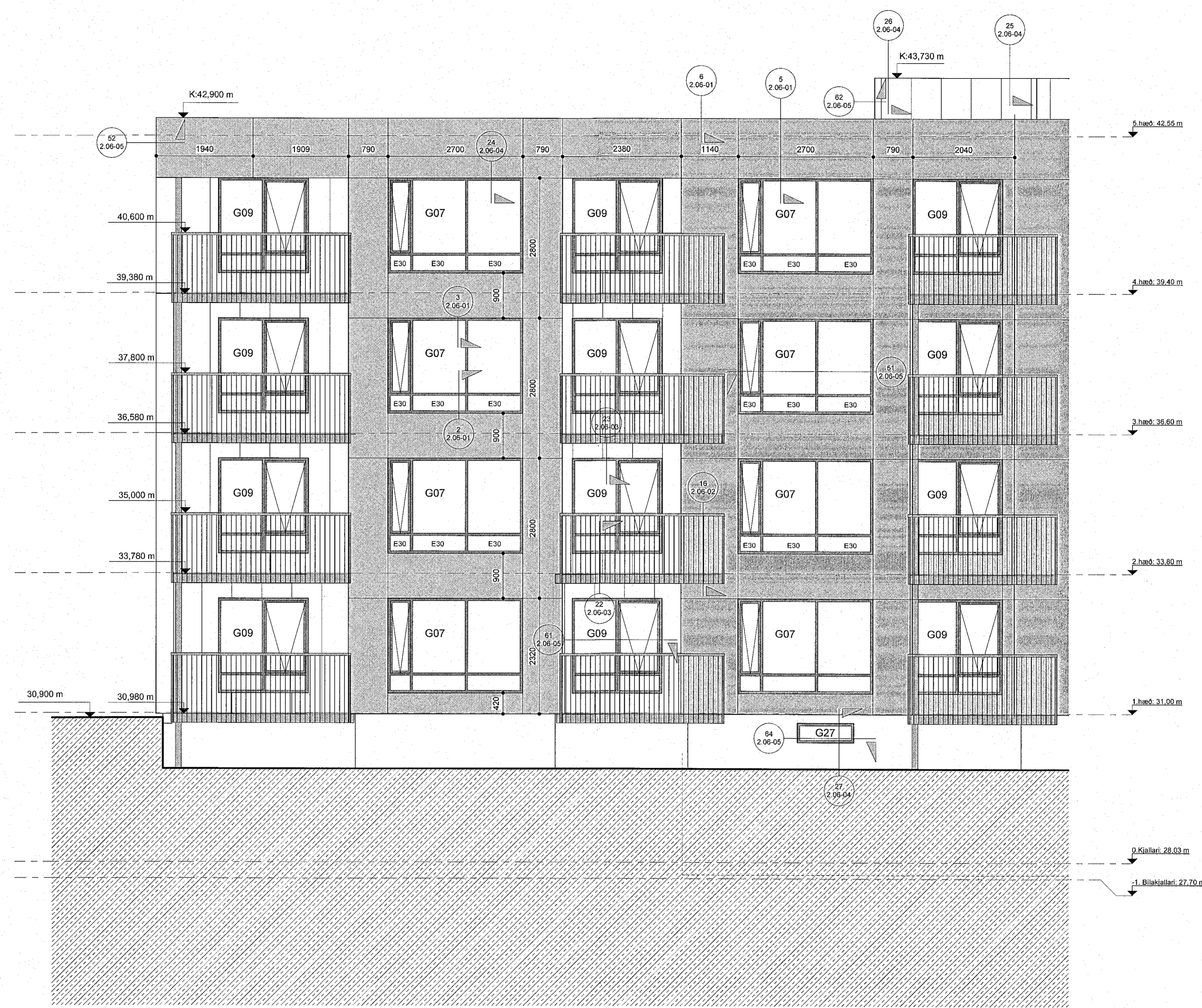
Áshamar 22 ásýnd vestur verkt. hluti 01 mkv: 1 : 50
