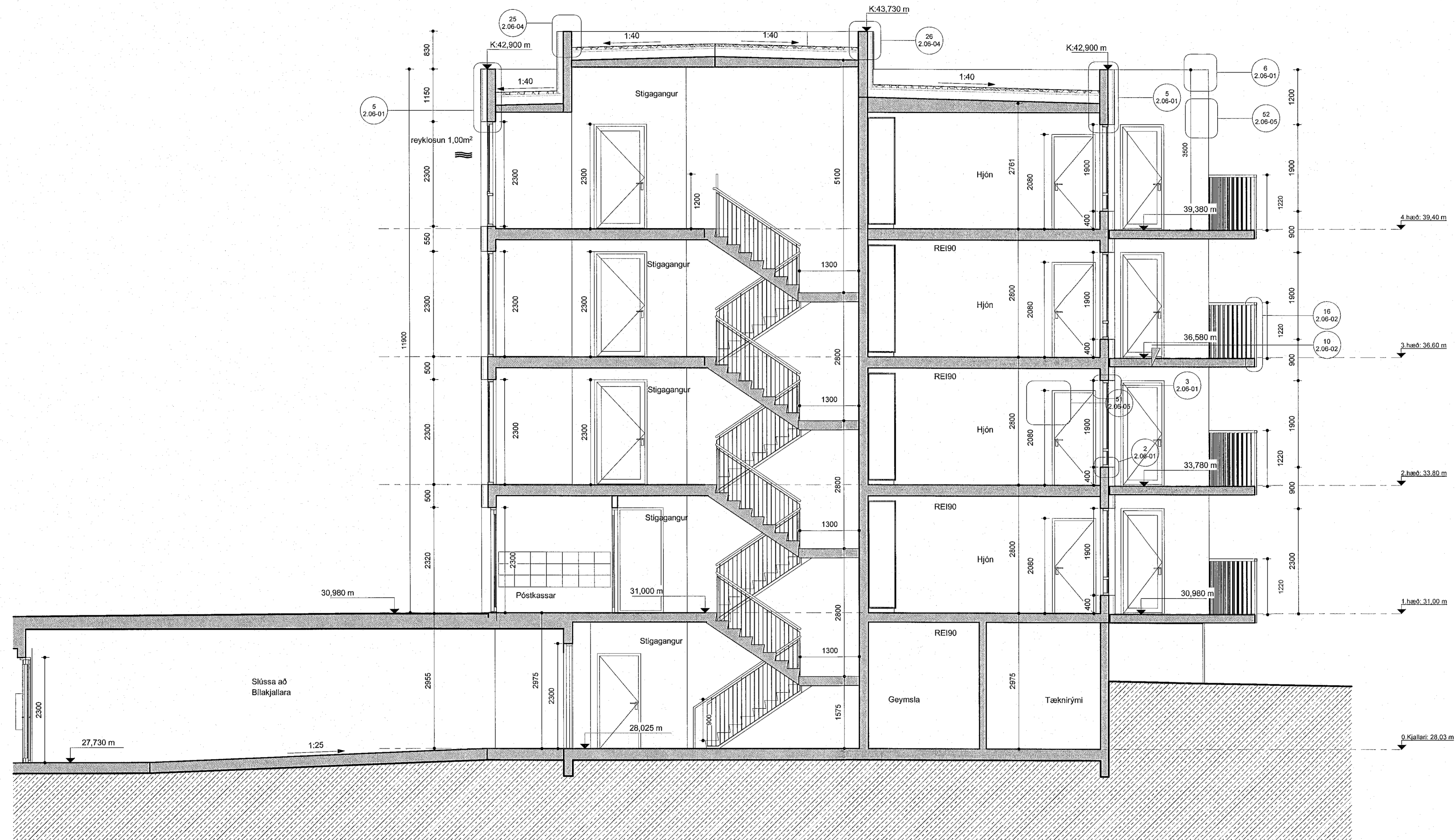
Áshamar 20 mhl.03 - snið e-e mkv: 1 : 50
