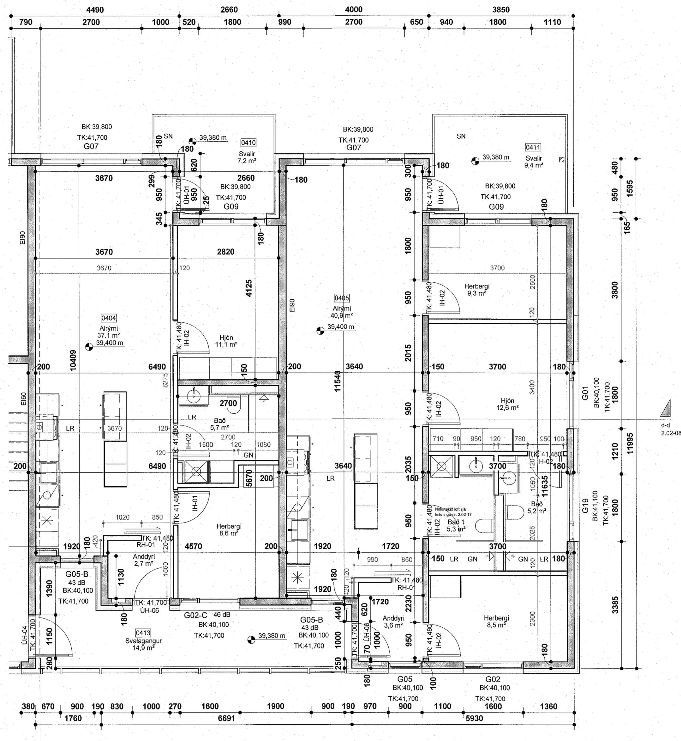
Áshamar 20 - 4.hæð - hluti 2 mkv: 1 : 50
