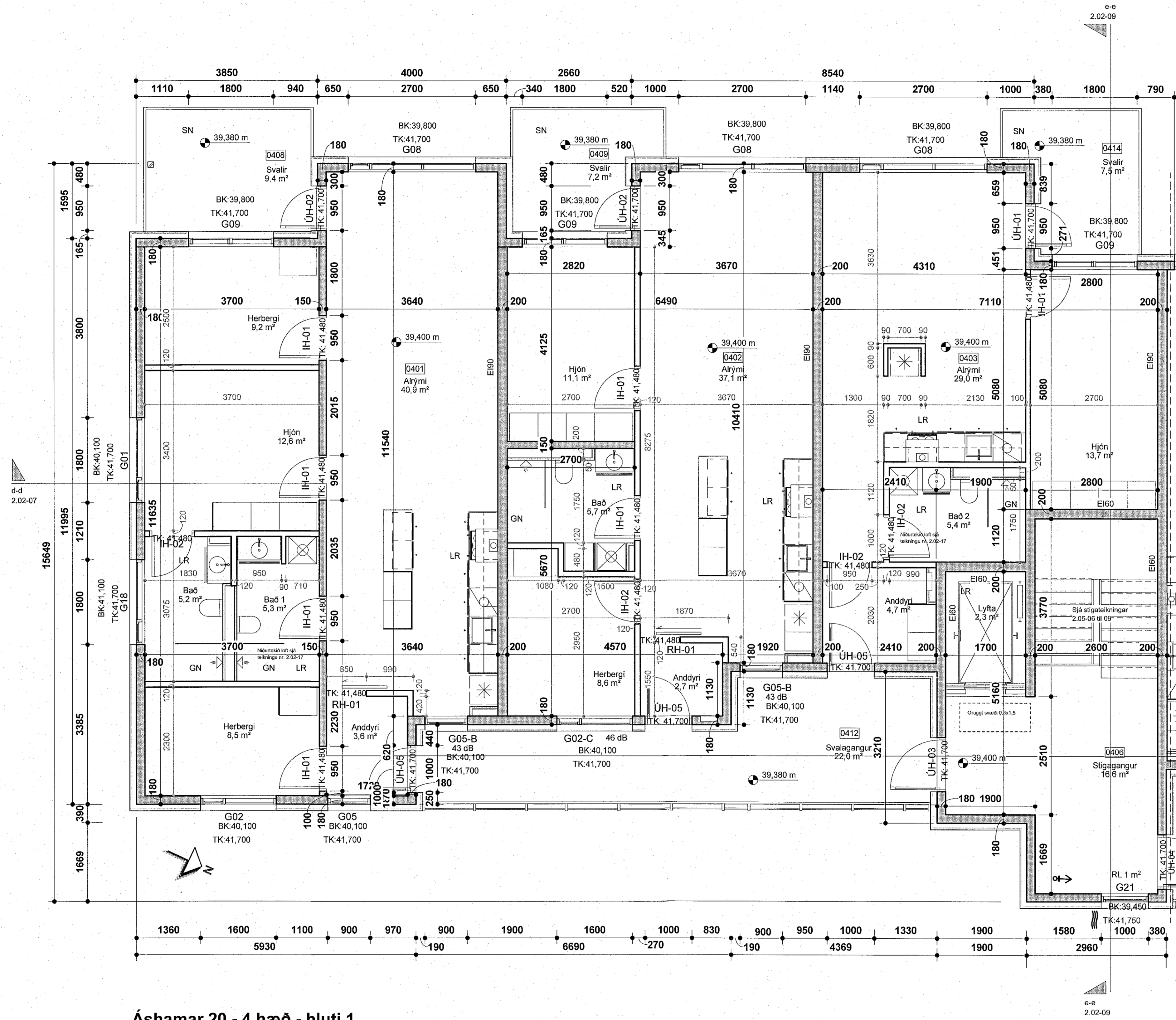
Áshamar 20 - 4.hæð - hluti 1 mkv: 1 : 50
