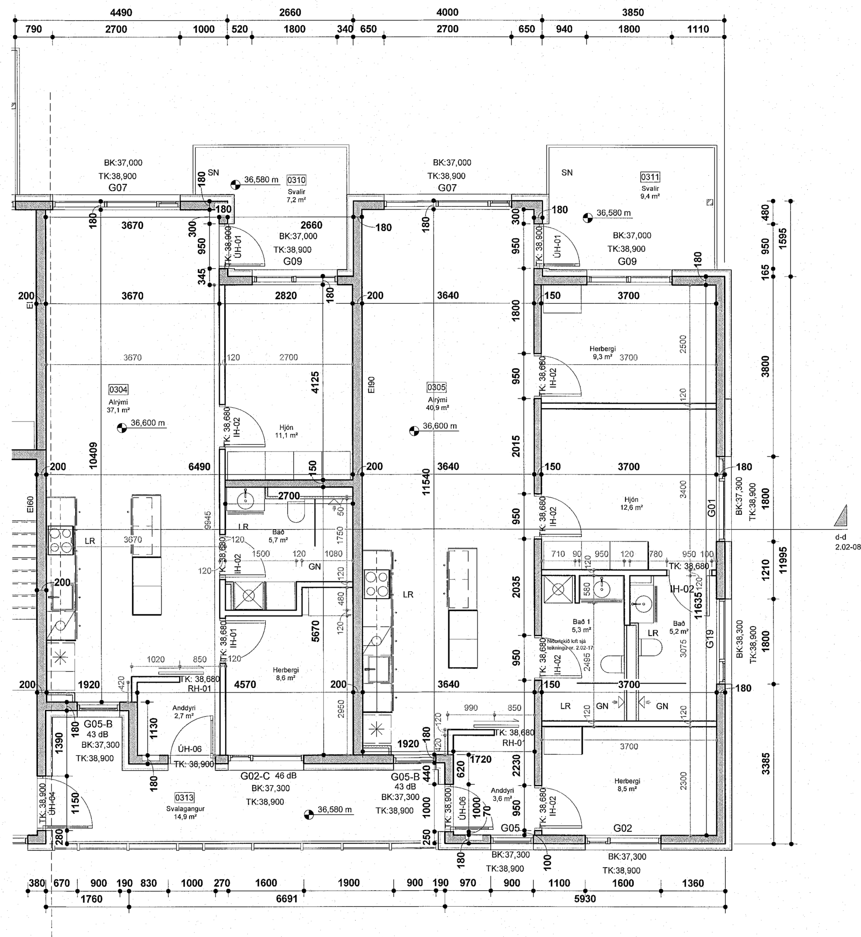
Áshamar 20 - 3.hæð - hluti 2 mkv: 1 : 50
