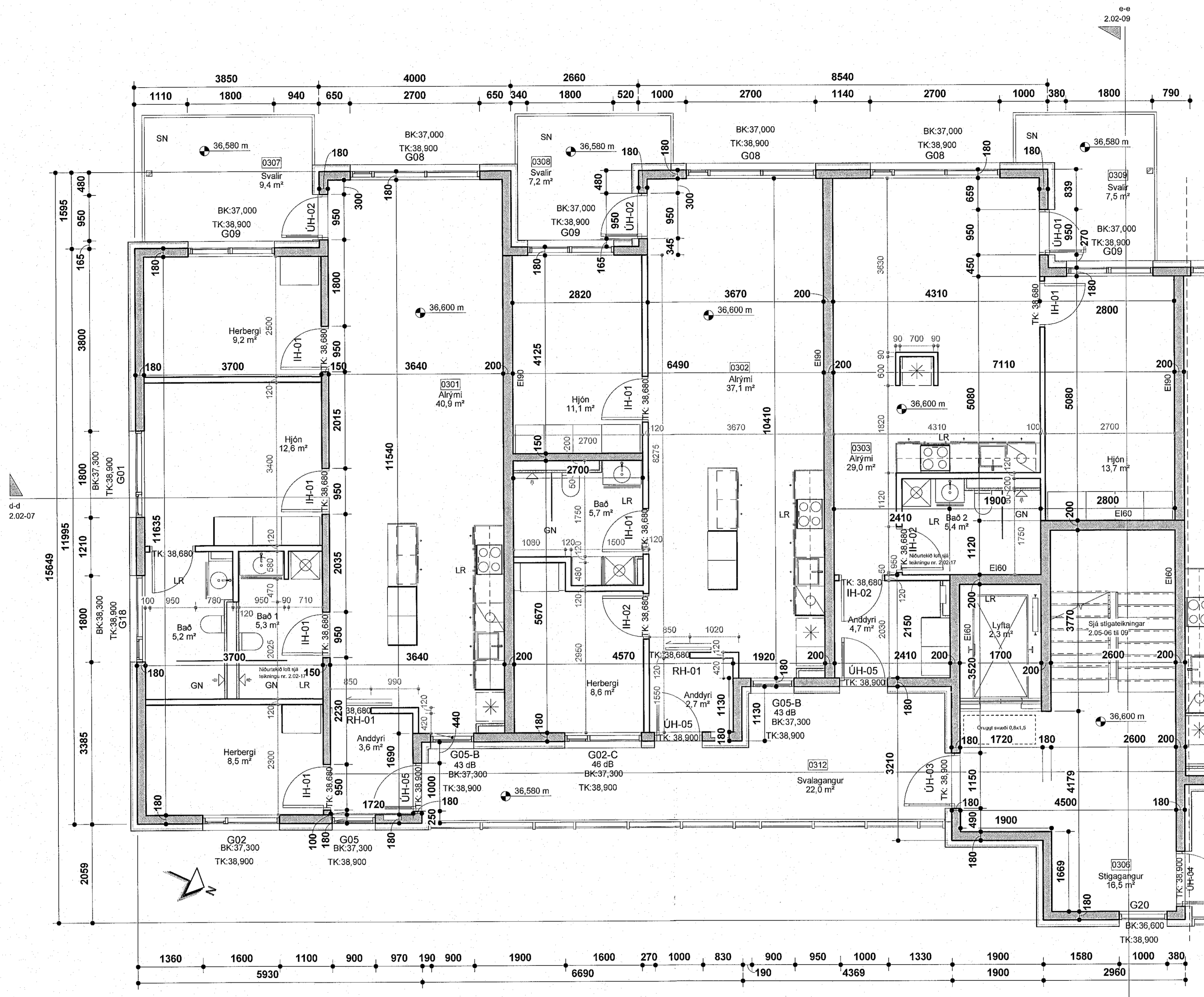
Áshamar 20 - 3.hæð - hluti 1 mkv: 1 : 50
