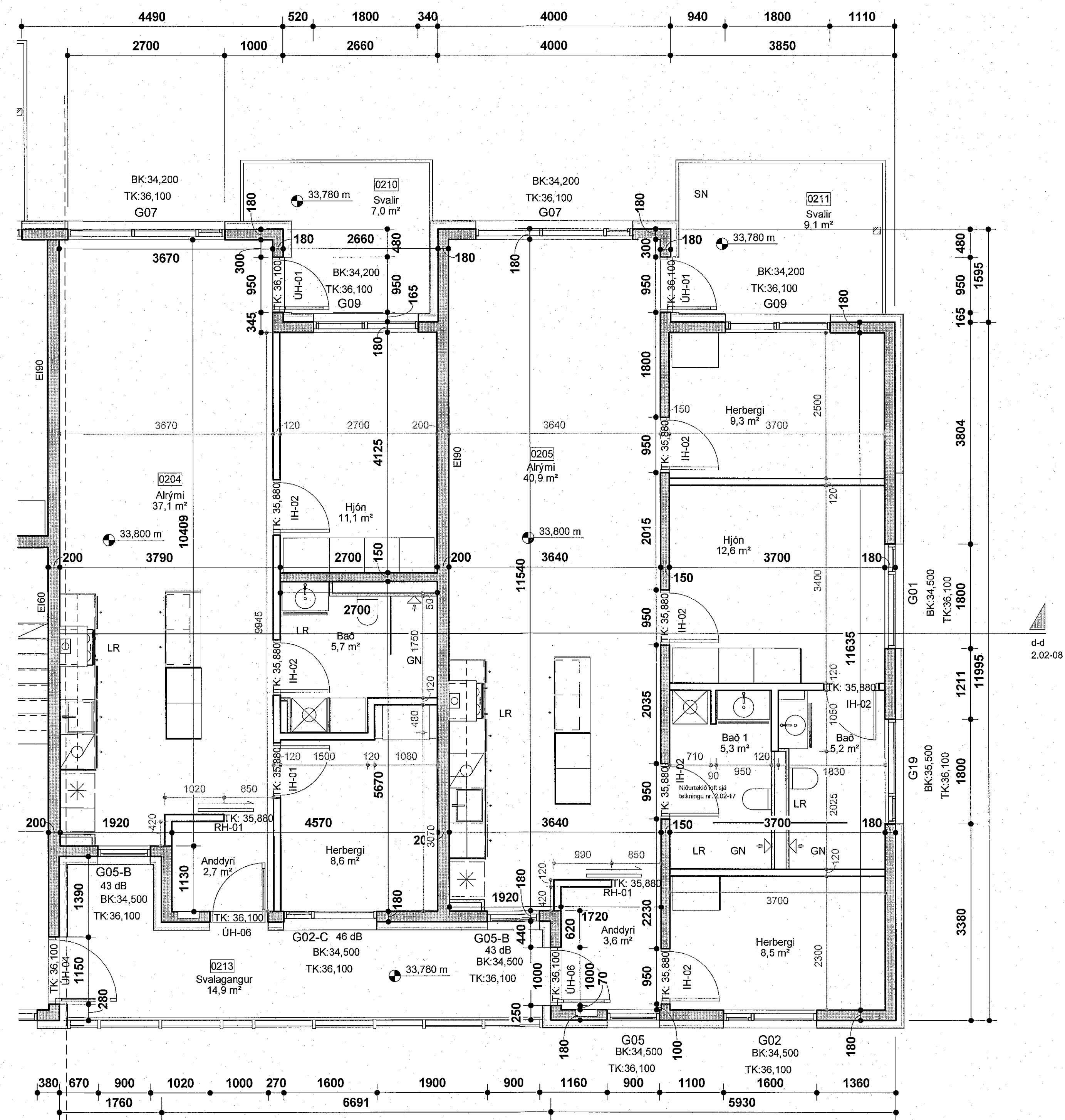
Áshamar 20 - 2.hæð - hluti 2 mkv: 1 : 50
