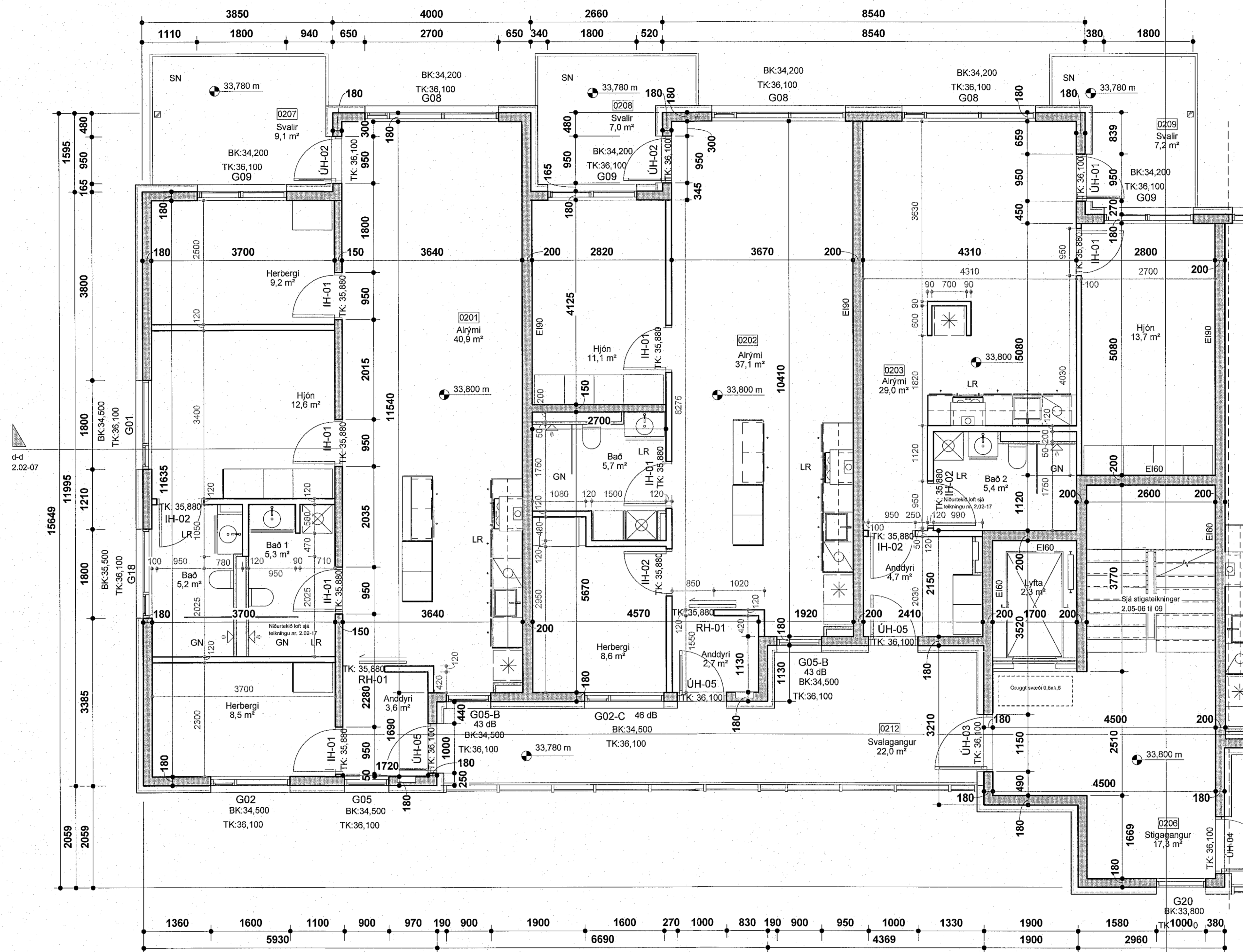
Áshamar 20 - 2. hæð - hluti 1 mkv: 1 : 50
