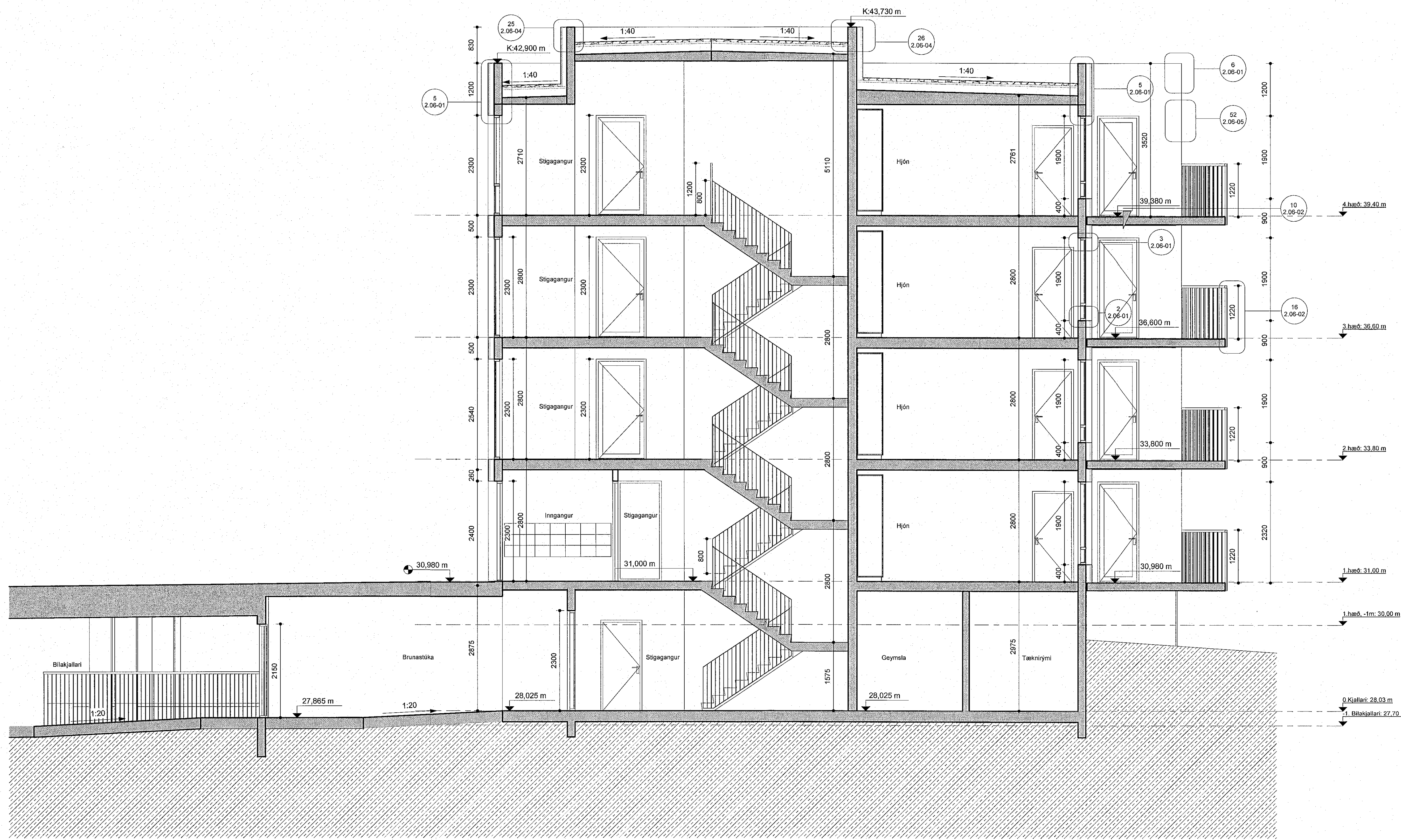
Áshamar 22- mhl.04 - snið f-f mkv: 1 : 50
