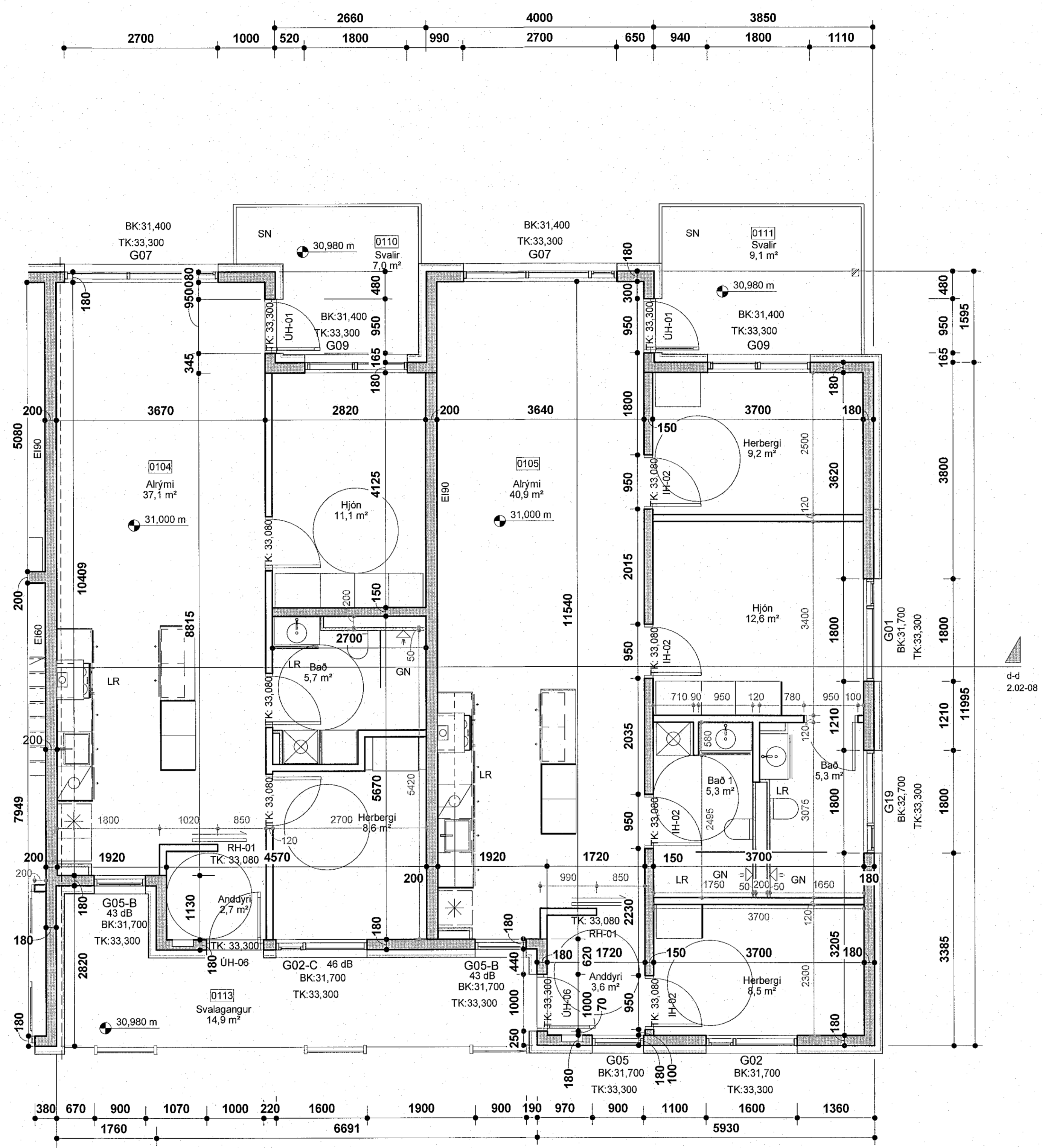
Áshamar 22 - 1. hæð - hluti 2 mkv: 1 : 50
