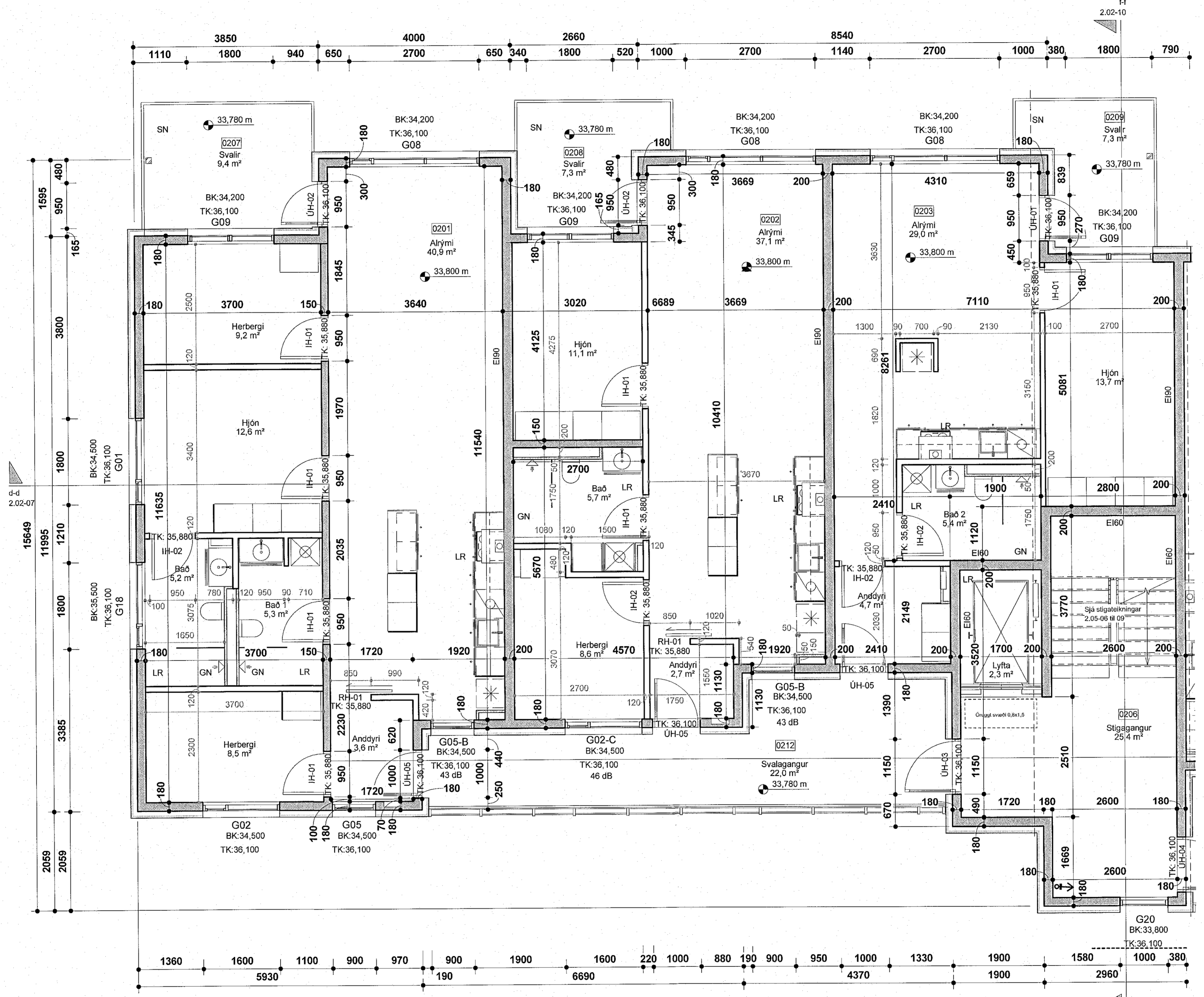
Áshamar 22 - 2.hæð - hluti 1 mkv: 1 : 50
