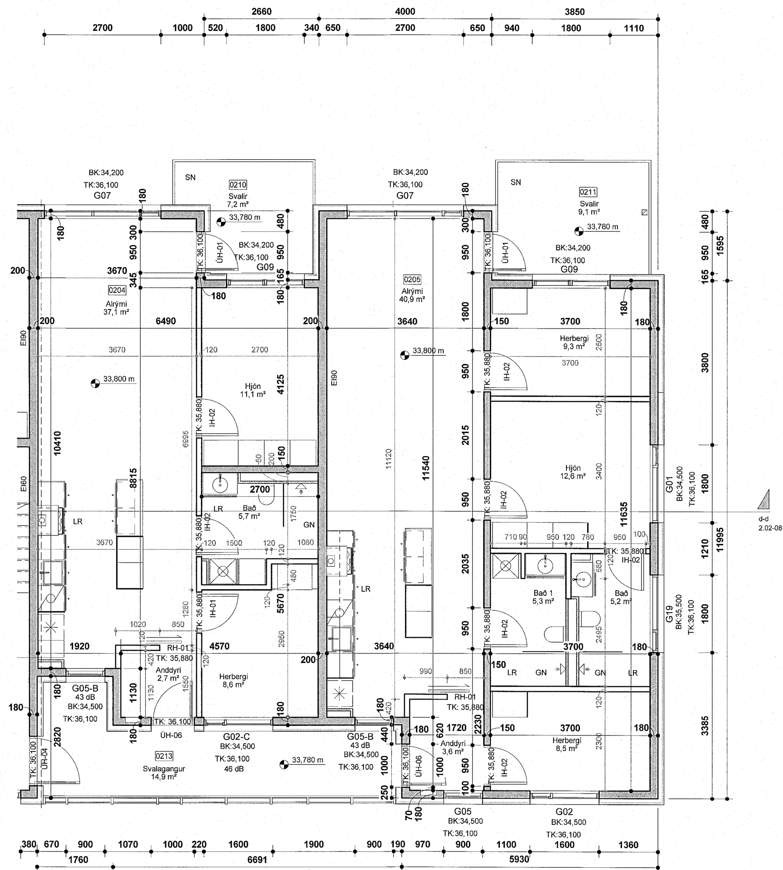
Áshamar 22 - 2. hæð - hluti 2 mkv: 1 : 50
