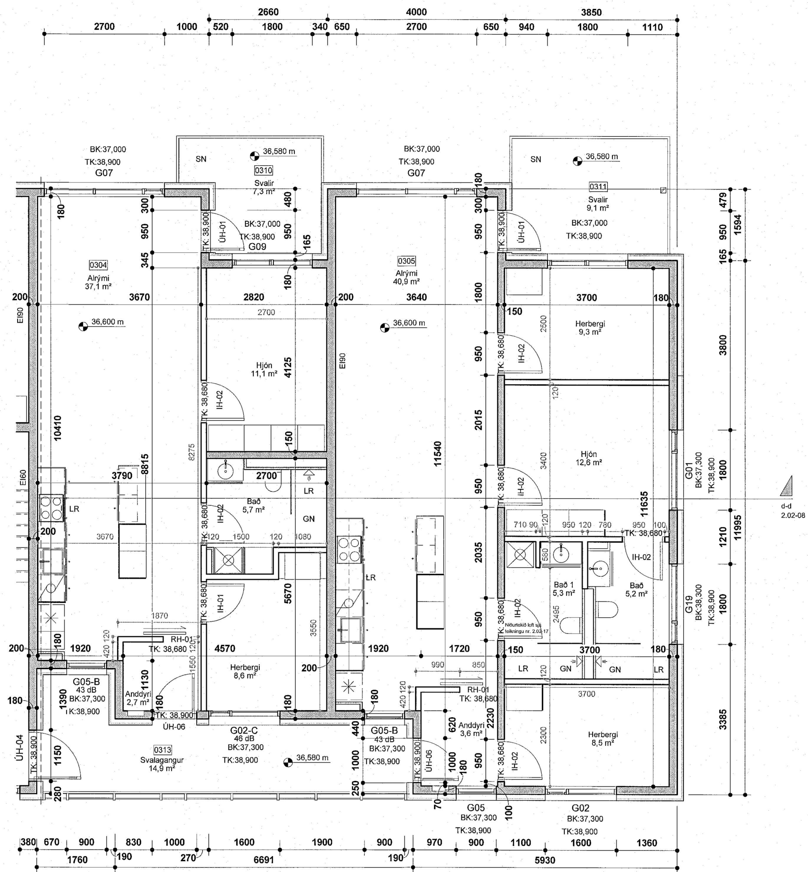
Áshamar 22 - 3. hæð - hluti 2 mkv: 1 : 50
