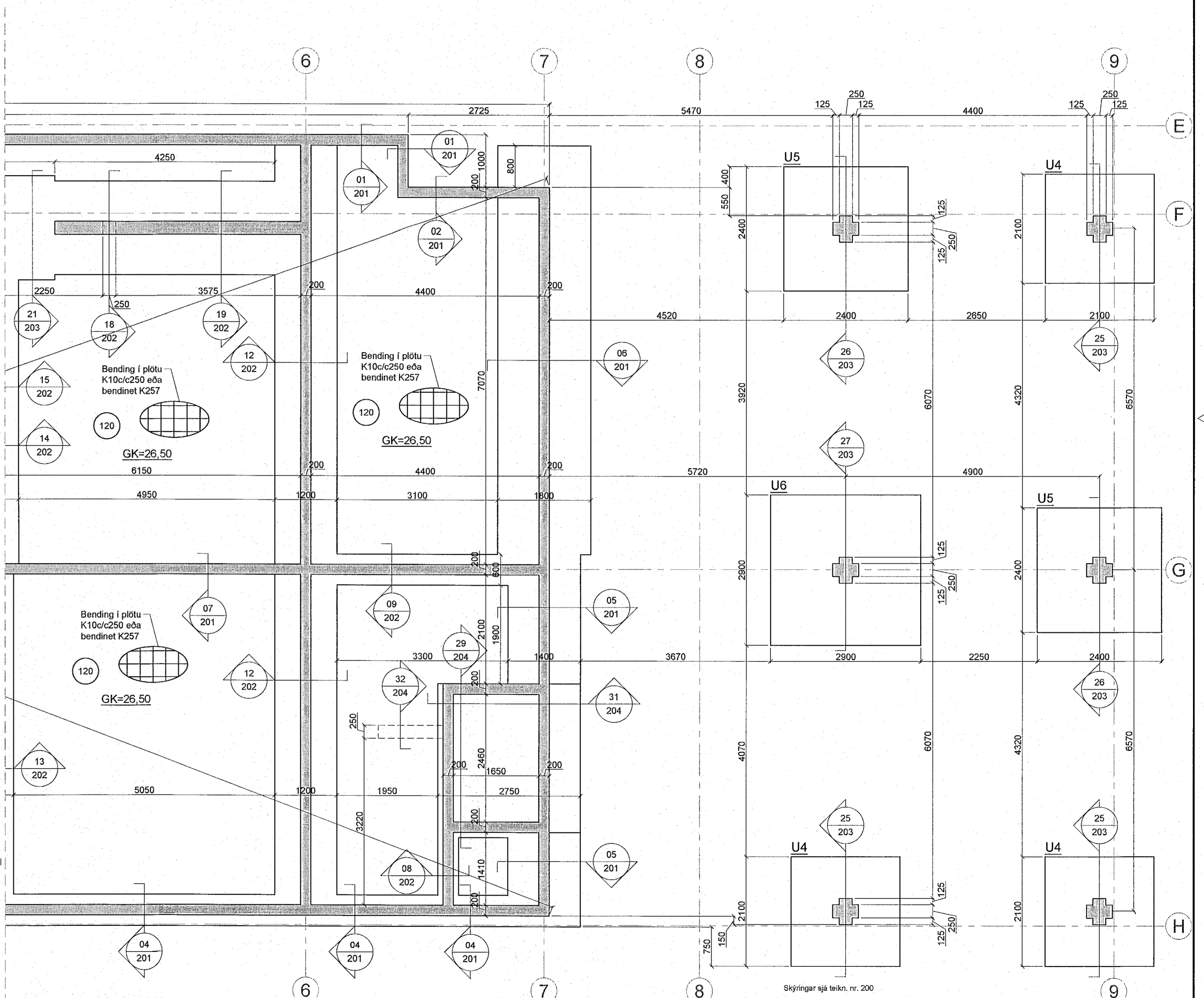
Grunnmynd sökkla, 1:50
