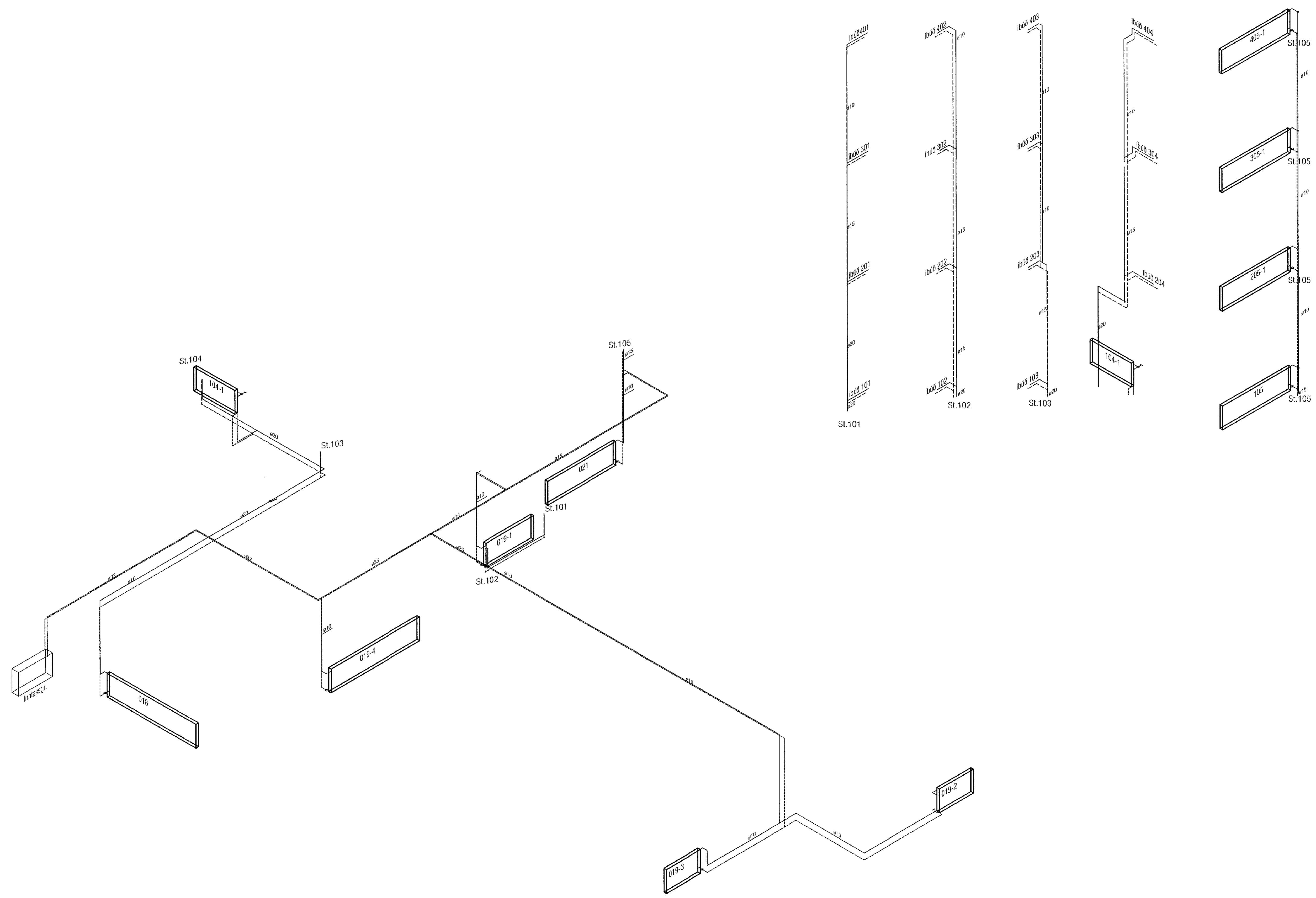
RÚMMYND OFNALAGNA LAGNIR ERU ÚR SVÖRTU STÁLI, SJÁ SKYRINGABLAÐ L-01
