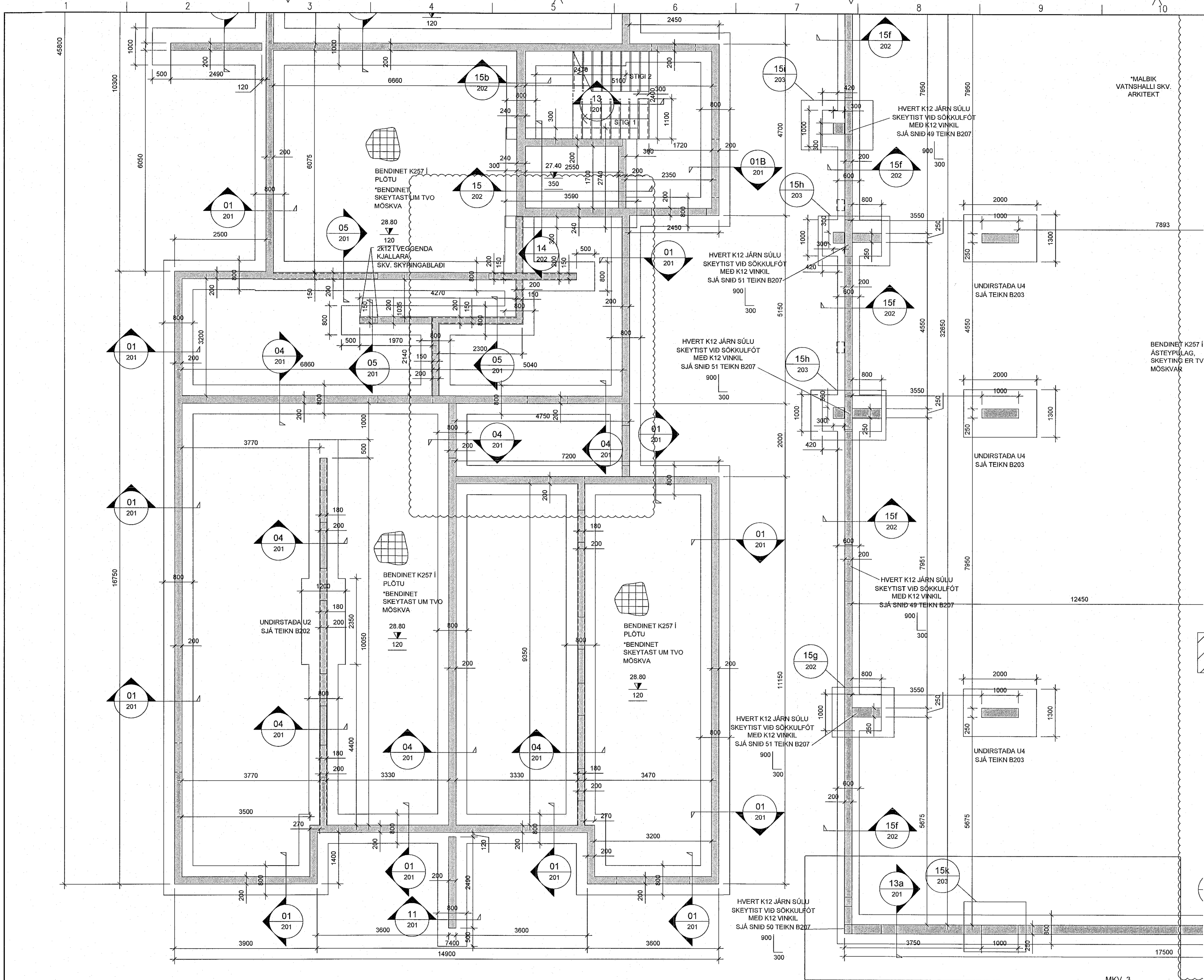
SÖKKLAR OG BOTNPLATA, GRUNNMYND MKV. 3
