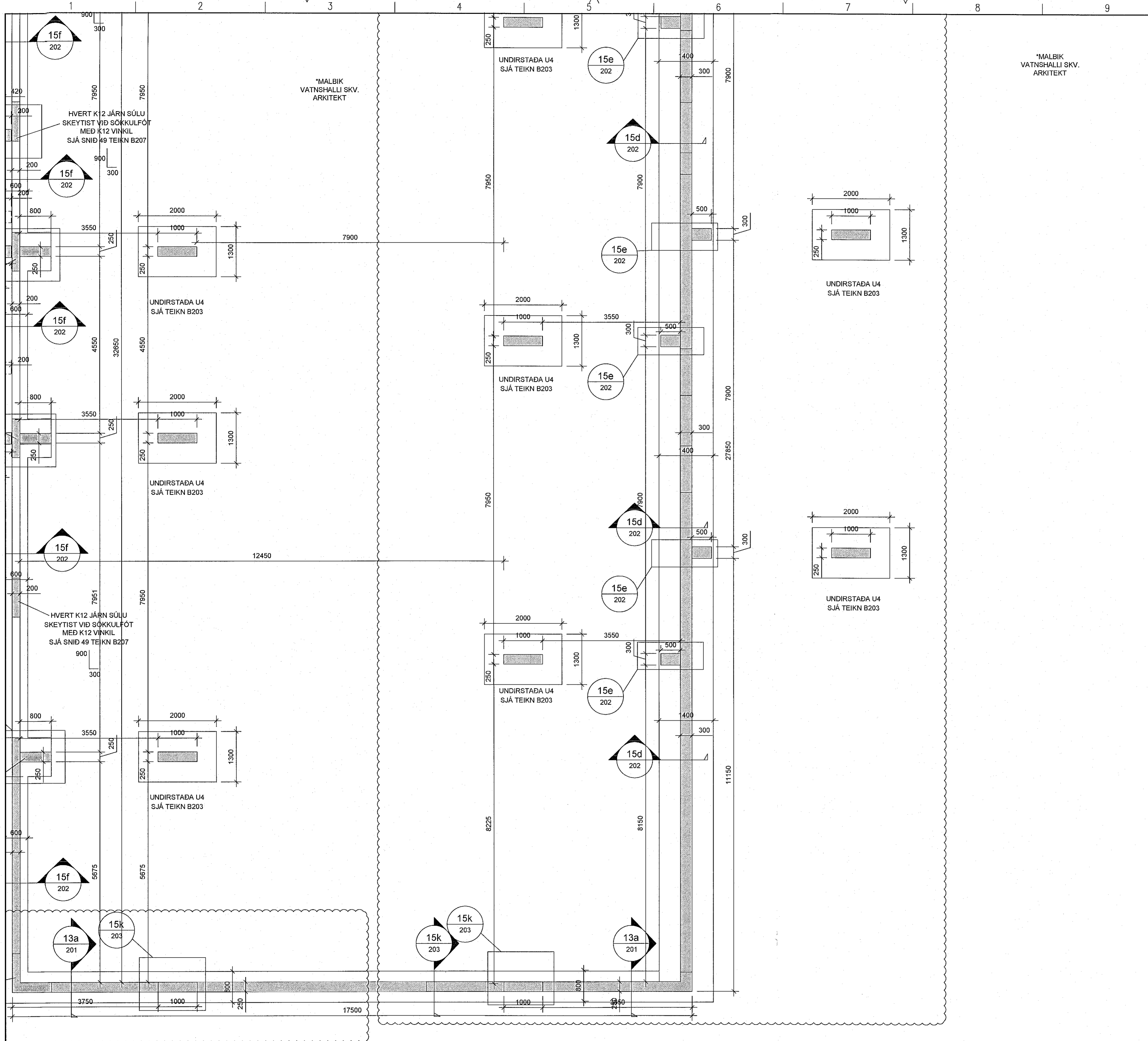
SÖKKLAR OG BOTNPLATA, GRUNNMYND MKV. 3
