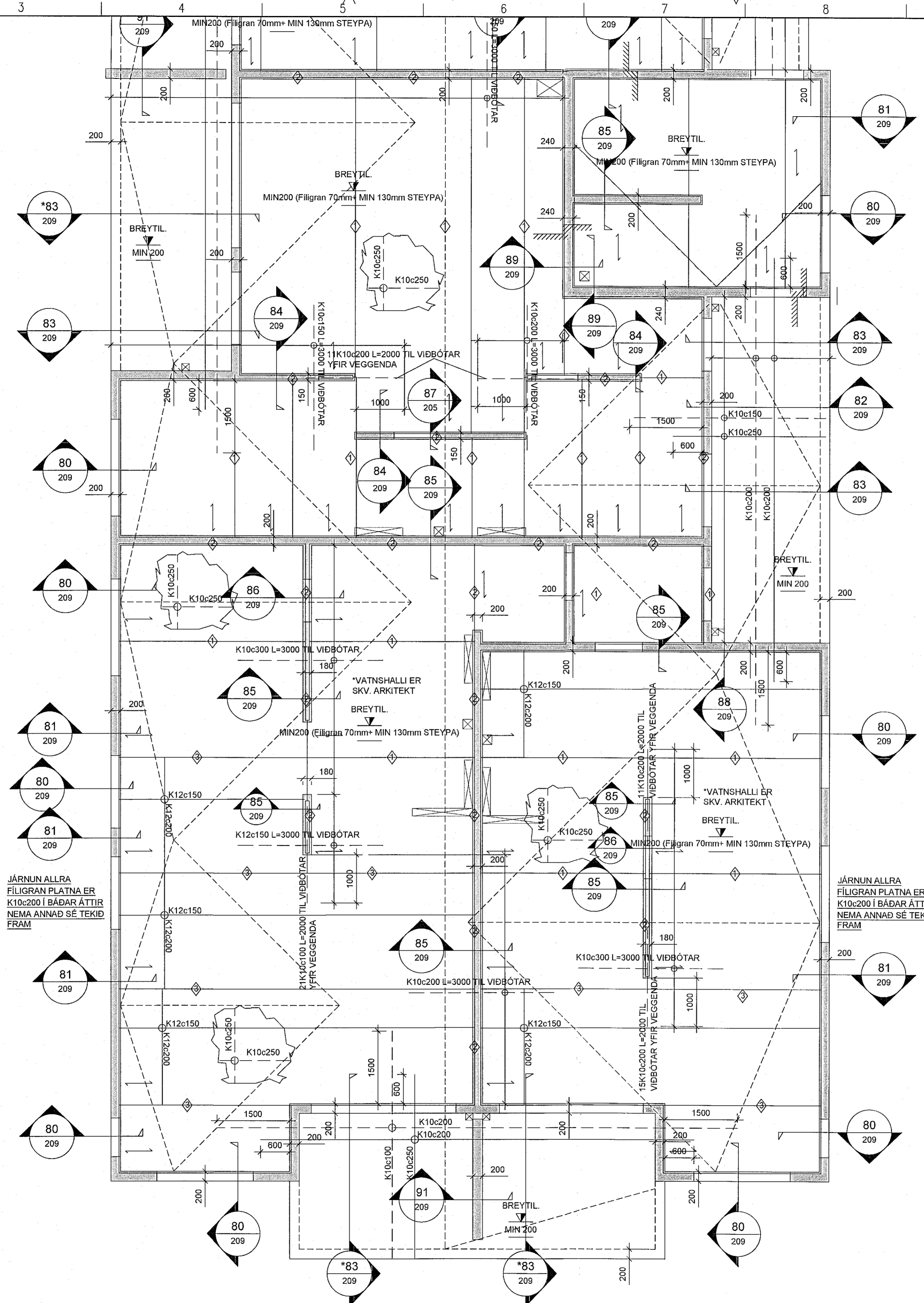
VEGGIR OG LOFTAPLATA 6.HÆÐAR, GRUNNMYND MKV. 3
