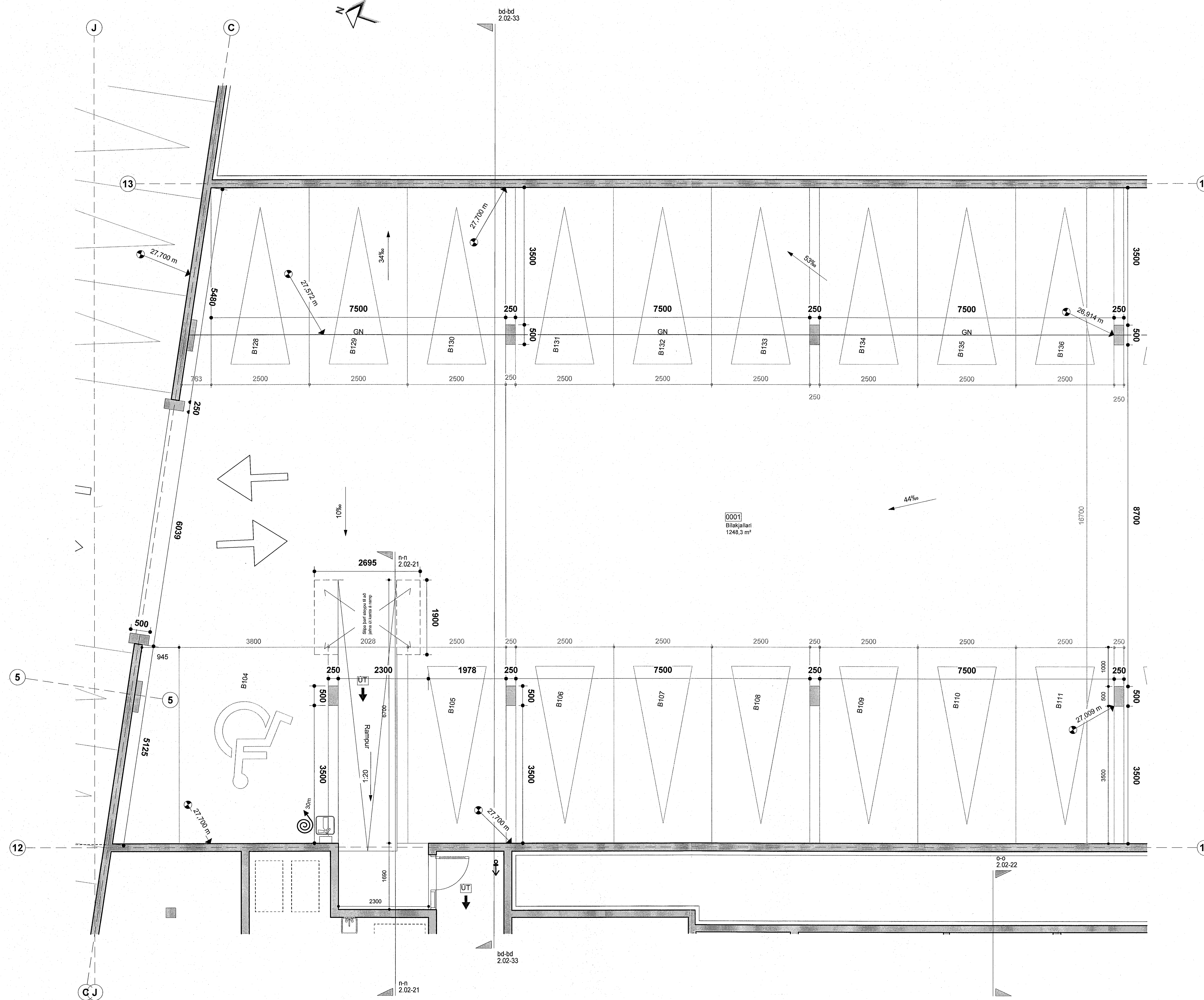
-1. Bílakjallari áfangi 2 - Hluti 1 mkv: 1 : 50
