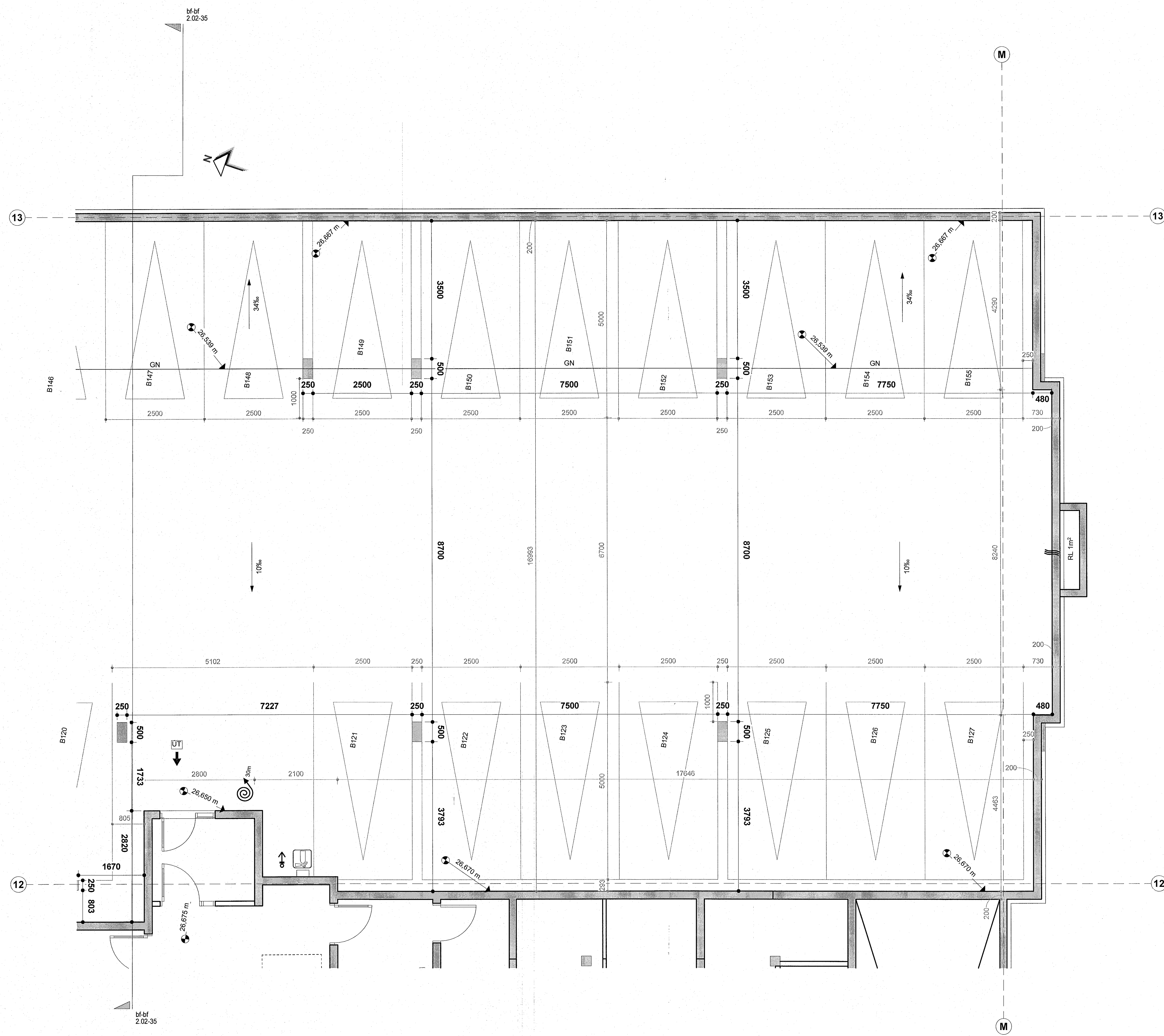
-1. Bílaskjallari áfangi 2 - Hluti 3 mkv: 1 : 50
