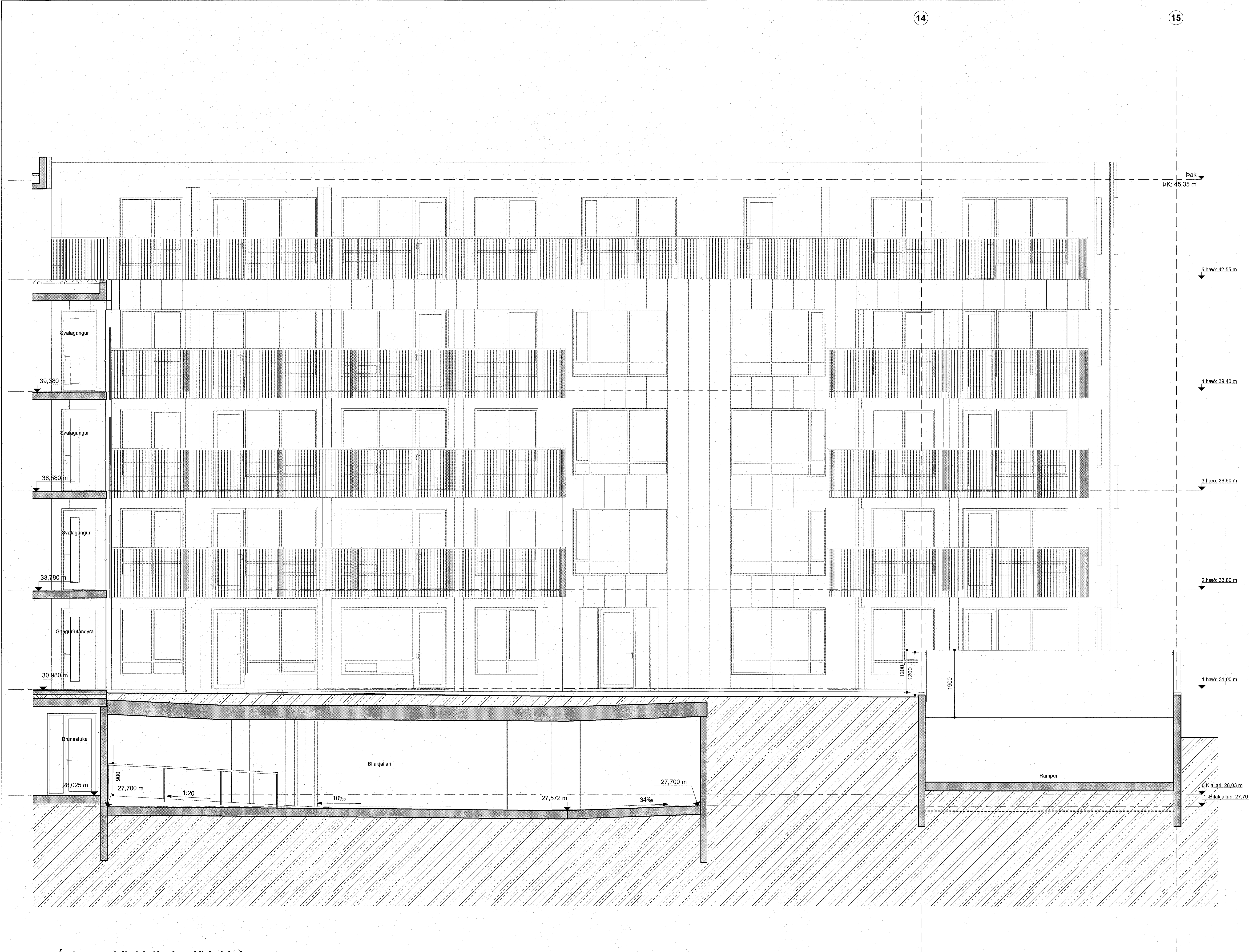
Áshamar bilakjallari snið bd-bd mkv: 1 : 50
