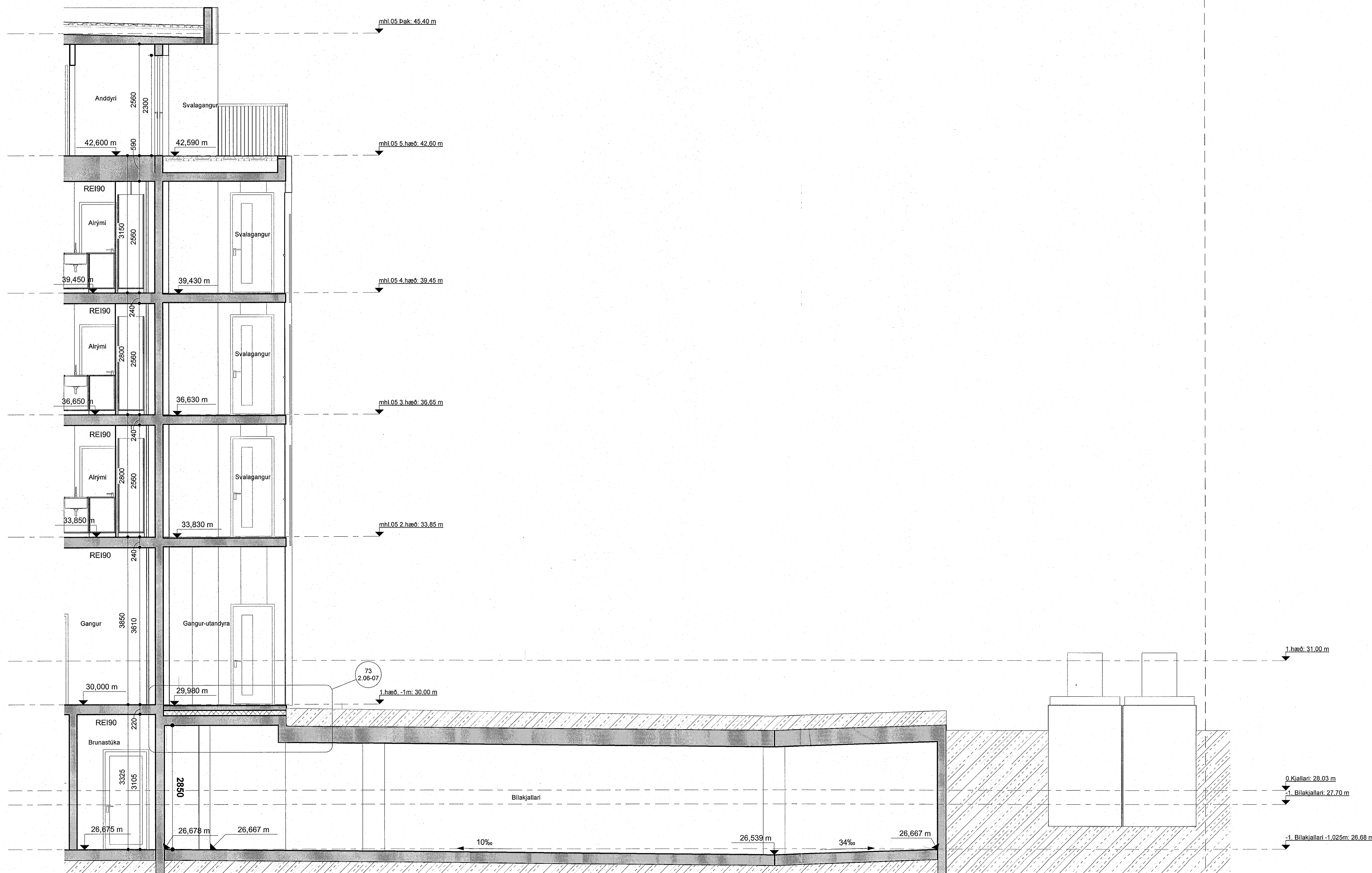
Ashamar bílakjallari snið bf-bf mkv: 1 : 50
