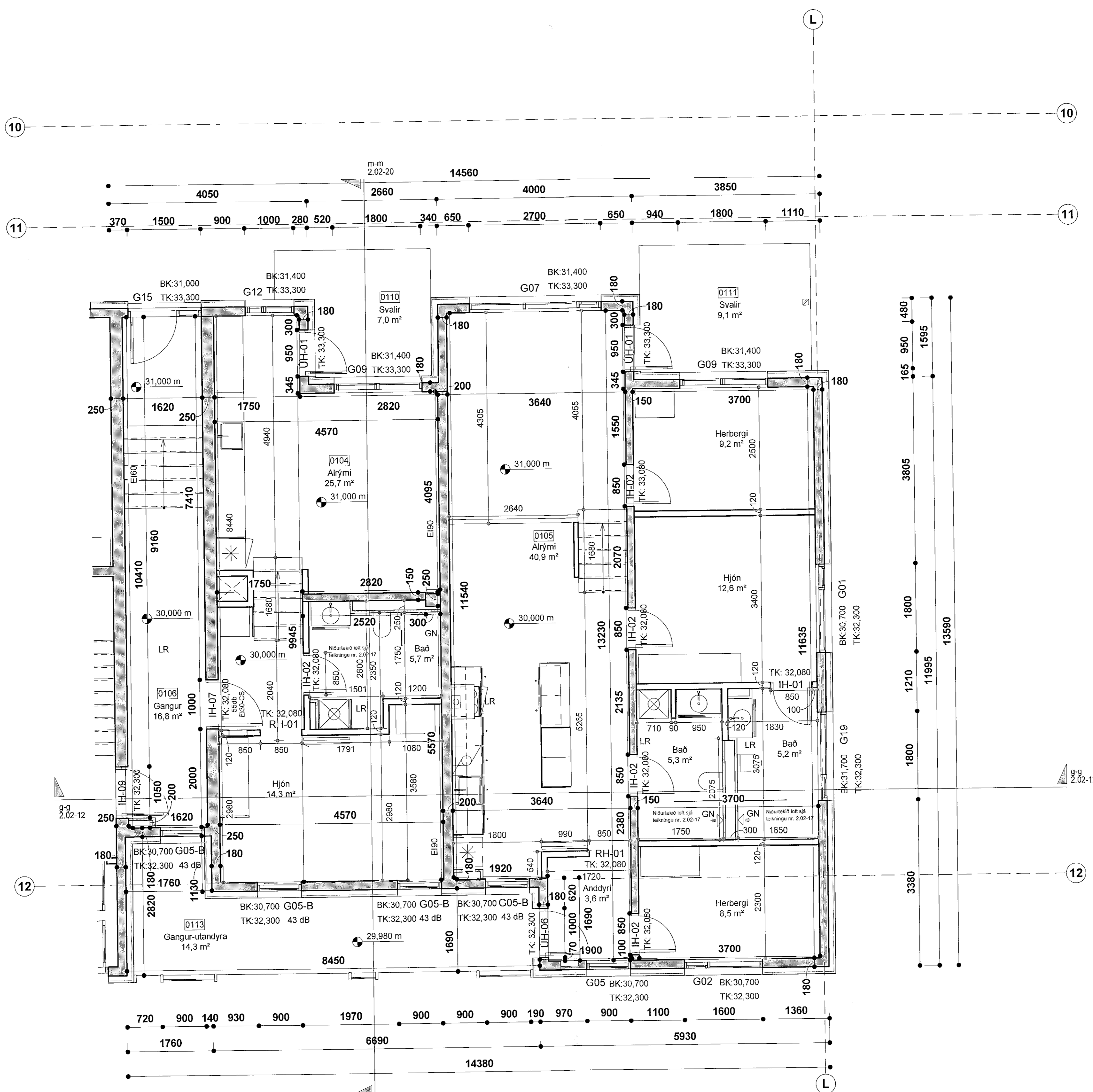
Áshamar 24 - 1.hæð - hluti 2 mkv: 1 : 50
