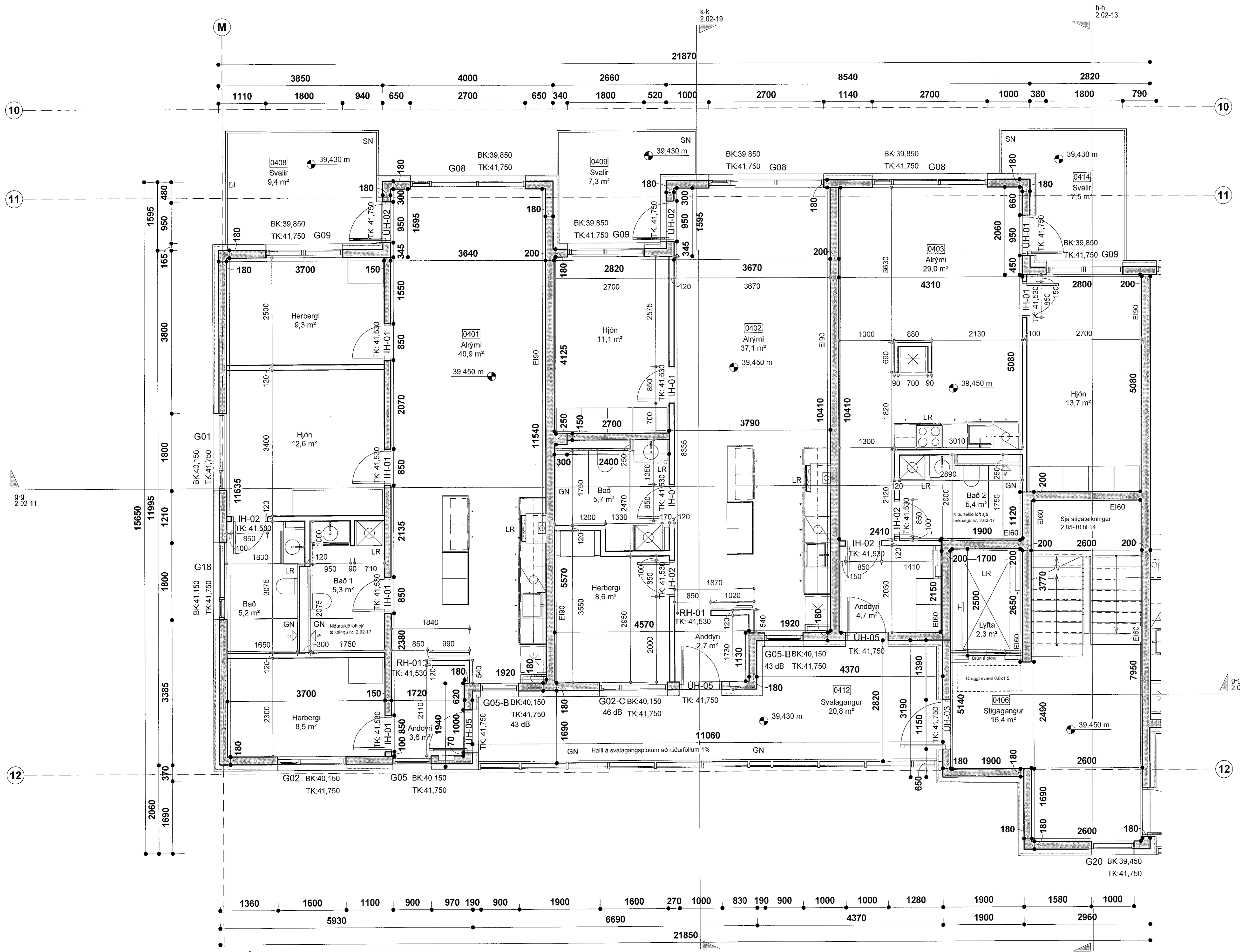
Áshamar 24 - 4.hæð - hluti 1 mkv: 1 : 50
