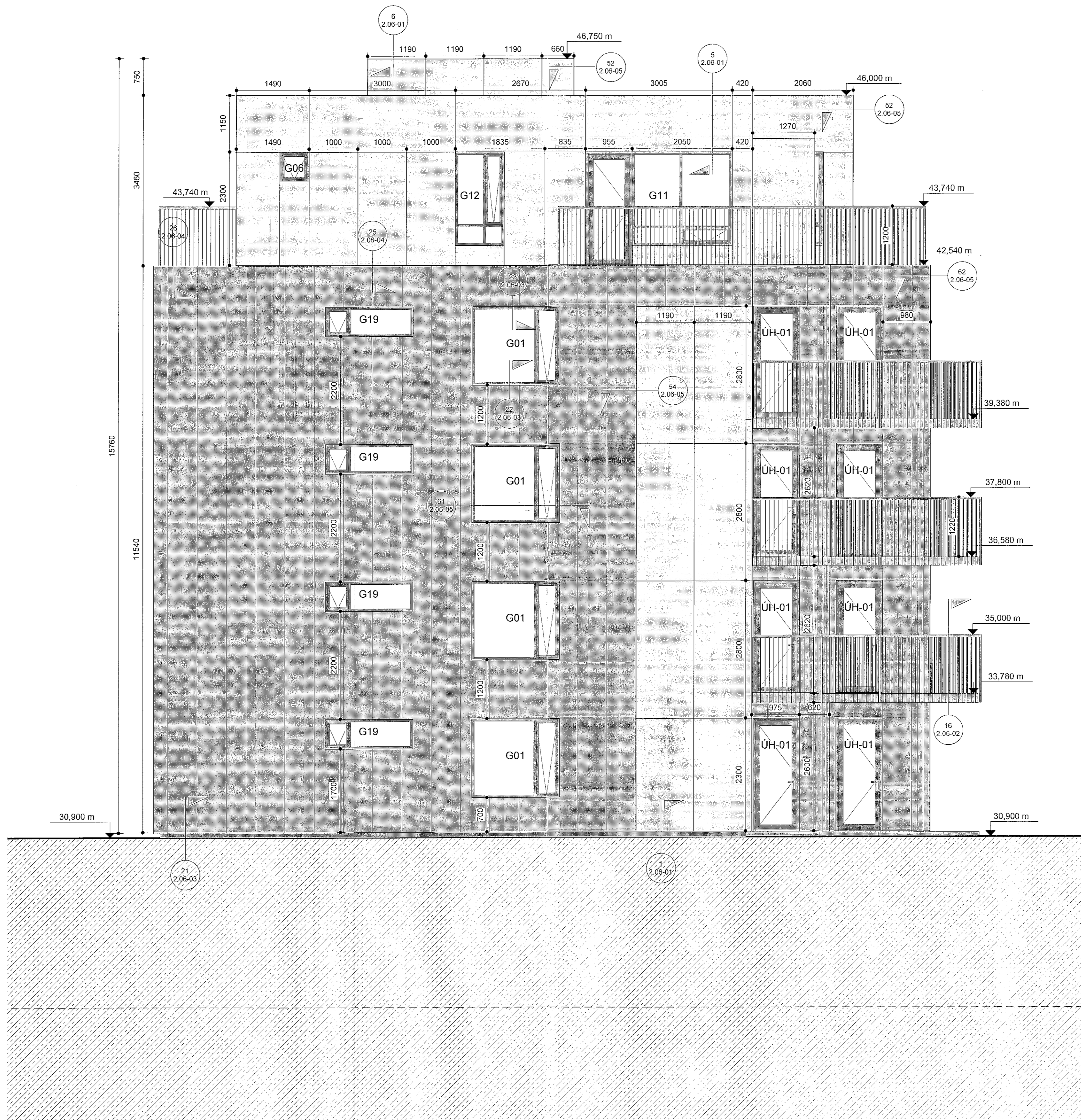
Áshamar 26 ásýnd norður verkt. mkv: 1 : 50
